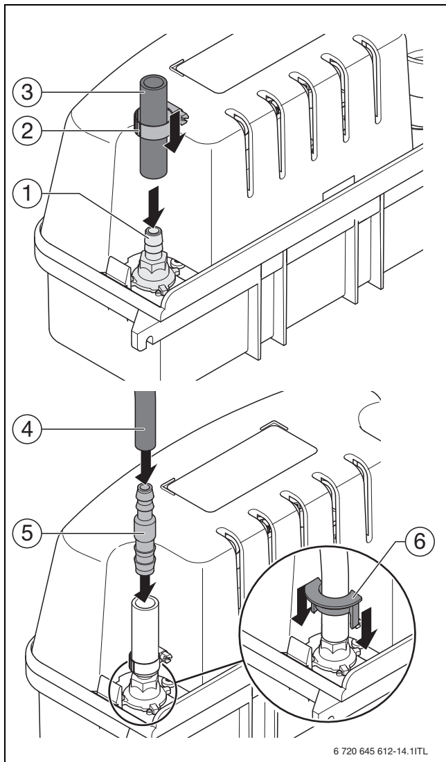
Afb. 9 Montage van de afvoerslang met adapter
