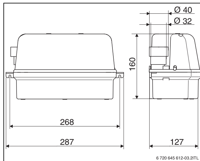
Fig. 2 Dimensiones
