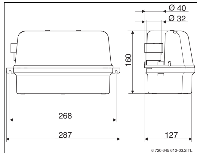
Fig. 2 Dimensioni
