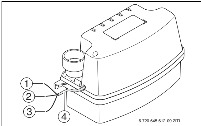
Bild 11 Drähte des Störungs-Anzeigesystems
