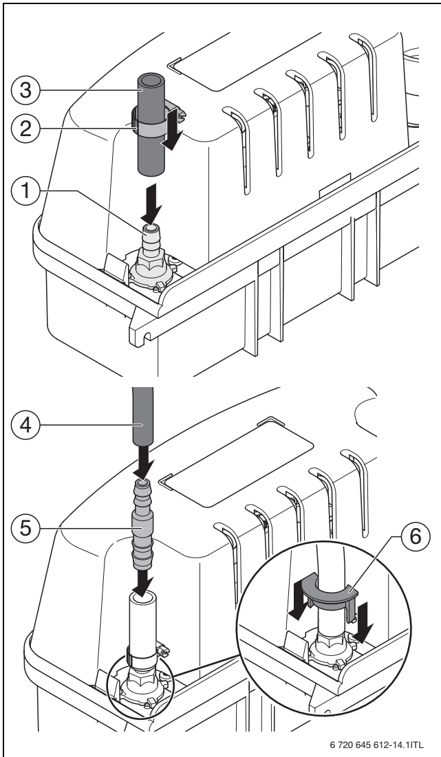
Bild 9 Ablaufschlauch mit Adapter montieren
