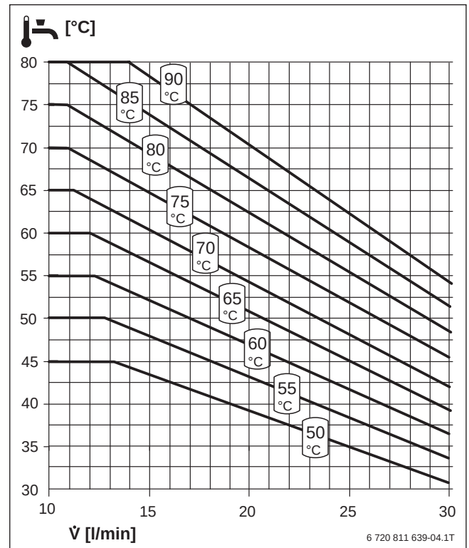
Bild 24 Temperaturverhalten FS/2
