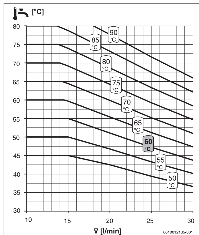
Bild 110 Temperaturverhalten FS20/2
