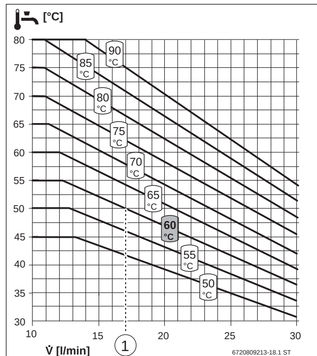
Bild 109 Temperaturverhalten FS/2
