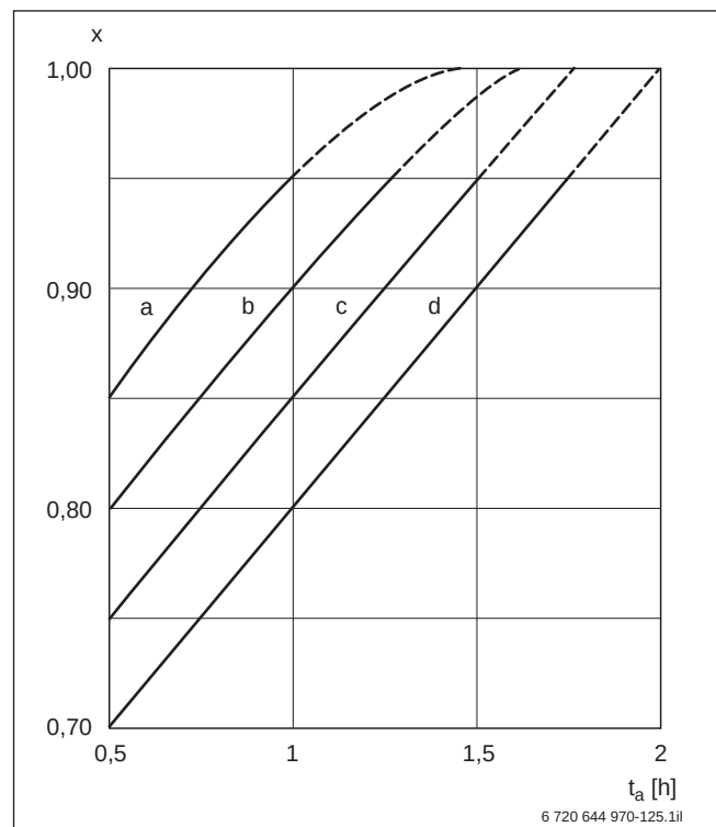
Bild 150 Übertragungs-Korrekturfaktor x
