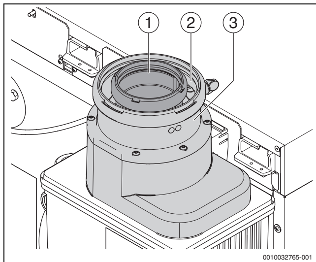
Bild 16 Abgasanschluss montieren
