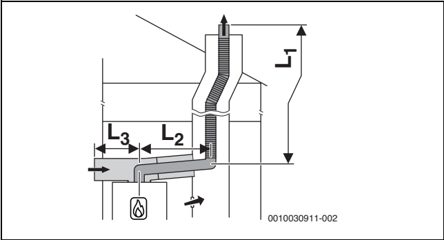
Bild 11 Flexible Abgasführung nach C 53x im Schacht und Luft-Abgas-Führung mit separater Luftzufuhr und konzentrischer Abgasableitung im Aufstellraum
