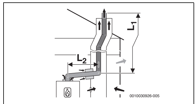
Bild 20 Flexible Abgasführung im Schacht nach B 53p mit raumluftabhängiger Luftzufuhr am Gerät und einwandiger Abgasleitung im Aufstellraum; Hinterlüftungsöffnung im Schacht
