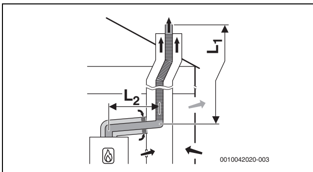
Bild 18 Flexible Abgasführung im Schacht nach B 53p /B 53S mit raumluftabhängiger Luftzufuhr über die konzentrische Verbindungsleitung im Aufstellraum; Hinterlüftungsöffnung im Schacht
