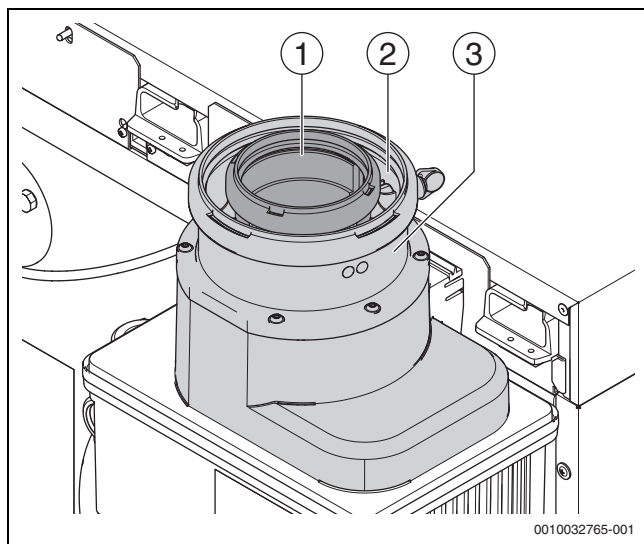
Bild 15 Abgasanschluss montieren
