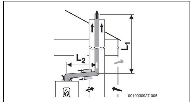
Bild 19 Starre Abgasführung im Schacht nach B 53p mit raumluftabhängiger Luftzufuhr am Gerät und einwandiger Abgasleitung im Aufstellraum; Hinterlüftungsöffnung im Schacht
