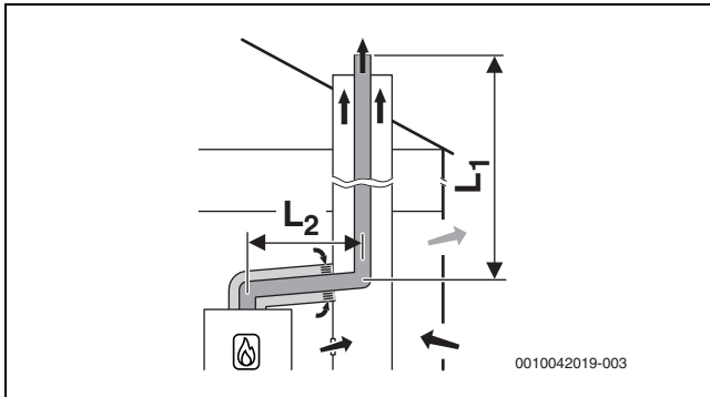
Bild 17 Starre Abgasführung im Schacht nach B 53p /B 53S mit raumluftabhängiger Luftzufuhr über die konzentrische Verbindungsleitung im Aufstellraum; Hinterlüftungsöffnung im Schacht
