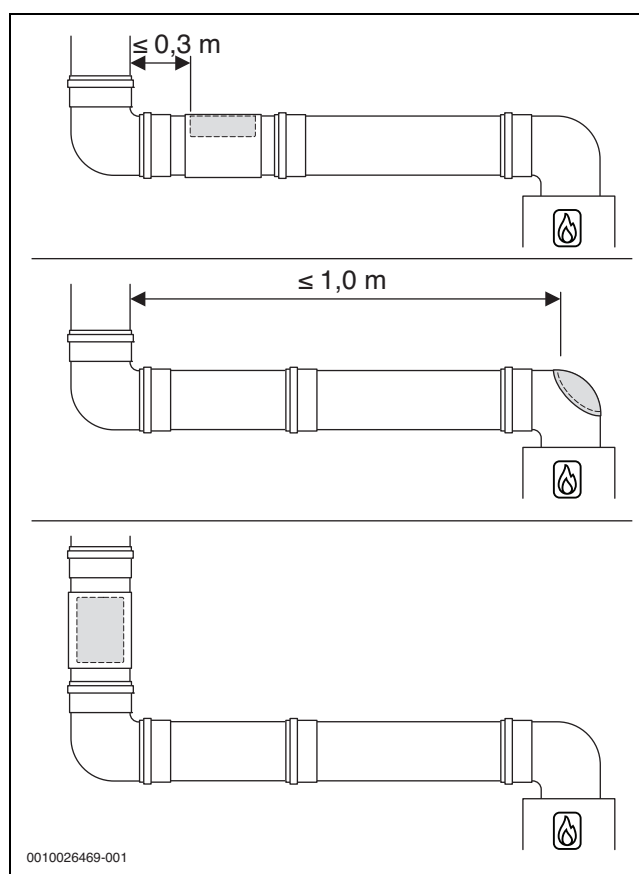
Bild 2 Anordnung der unteren Prüföffnung
