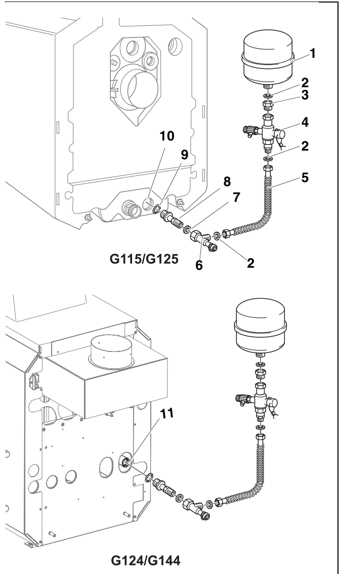
Abb. 1 Ausdehnungs- und Entleerungs-Set montieren
