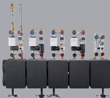
Logaflow HS40 / HS50 HKV2 / HKV3 für zwei und drei Heizkreise
