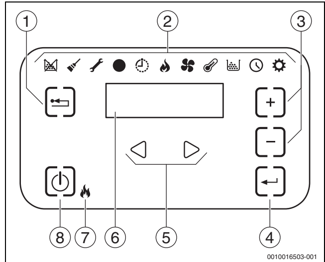
Bild 8 Bedienfeld
