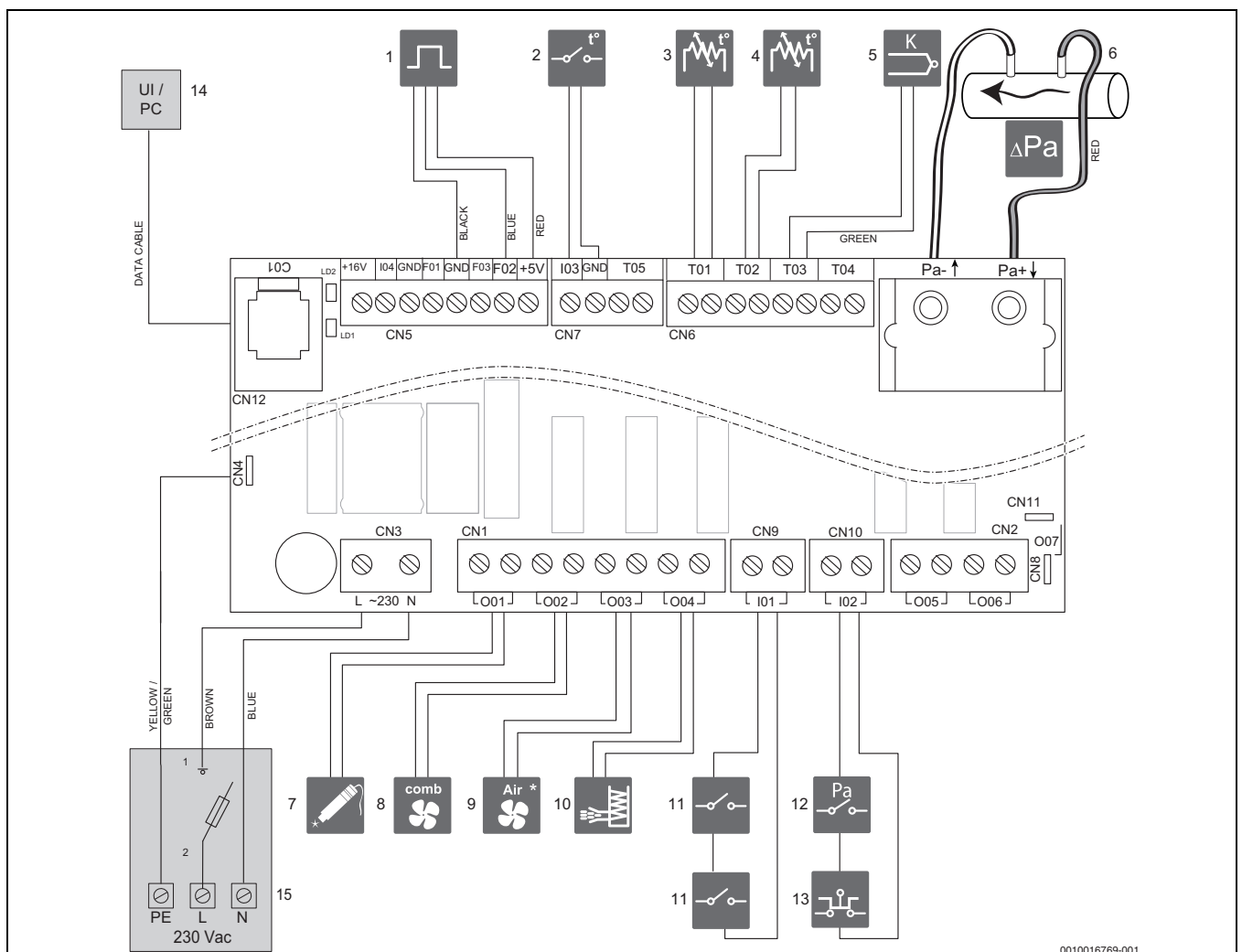
Bild 10 Anschlussplan
