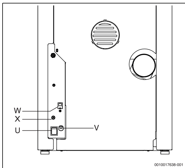
Bild 9 Anschlüsse Rückseite
