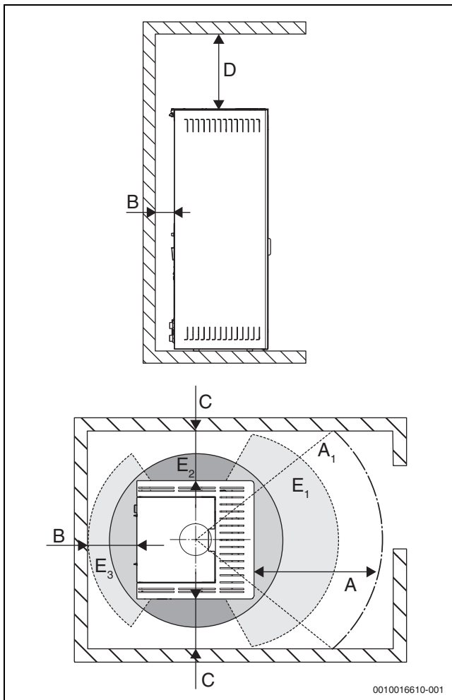
Bild 5 Mindestabstände
