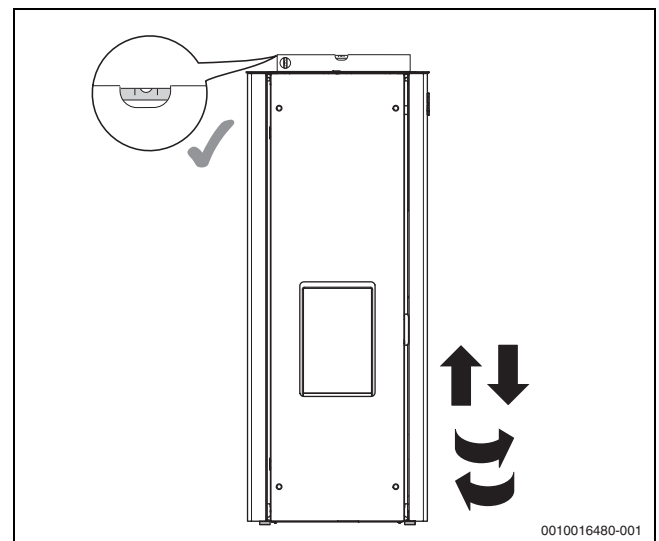
Bild 6 Ofen ausrichten
