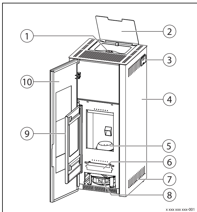
Bild 3 Produktübersicht
