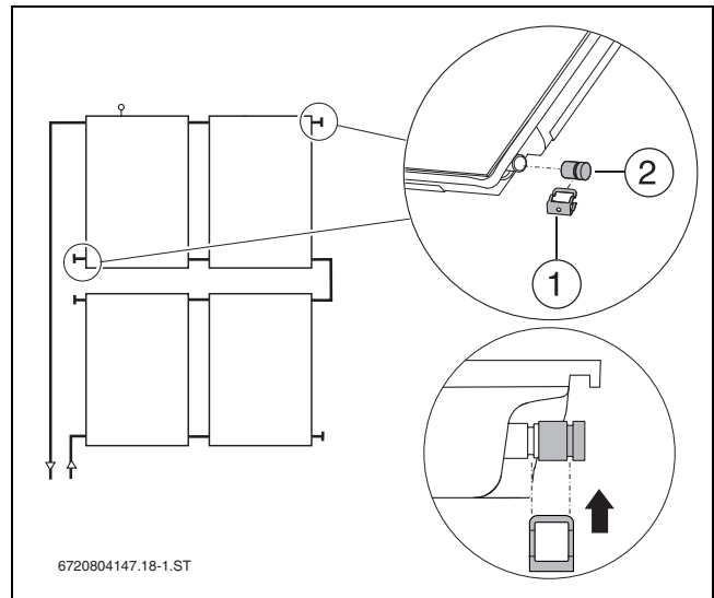
Bild 66 Kappen montieren
