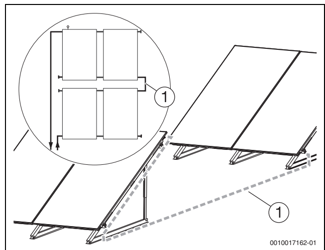
Bild 67 Verbindung zwischen den Kollektorreihen herstellen
