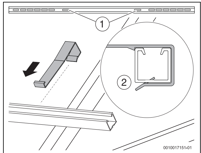
Bild 45 Abrutschsicherung an Profilschiene unten montieren
