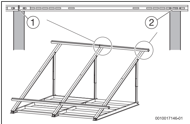
Bild 41 Profilschienen positionieren
