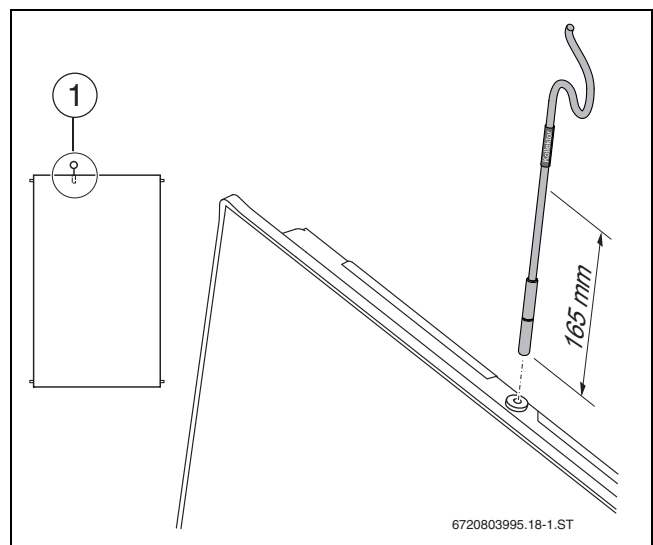
Bild 59 Kolleortemperaturfühler montieren
