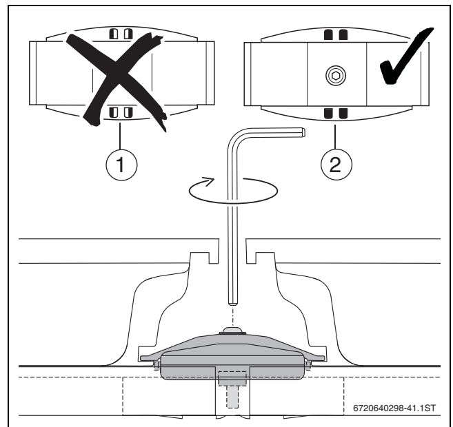
Bild 55 Kollektorspanner montiert
