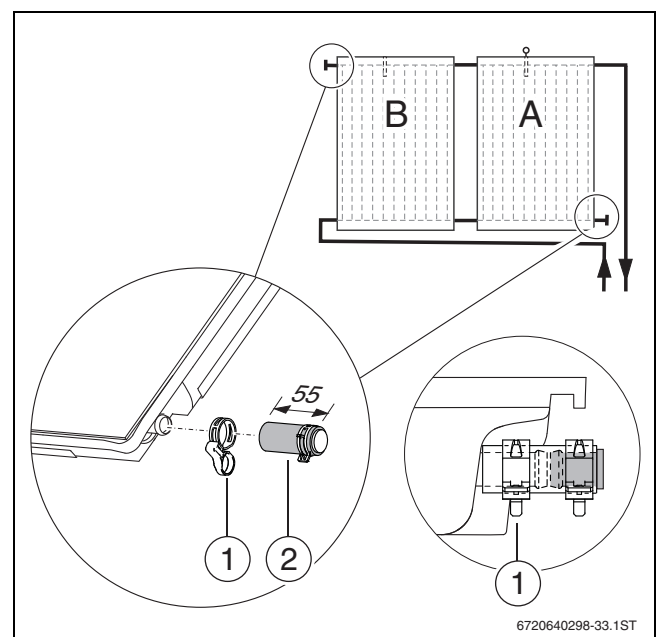
Bild 48 Stopfen montieren
