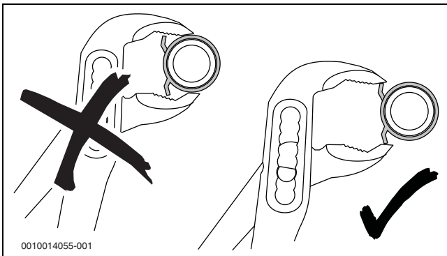
Bild 46 Federbandschelle ohne Sicherungsring versetzen
