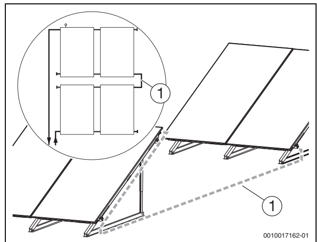
Bild 67 Bauseitige Rohrleitung montieren
