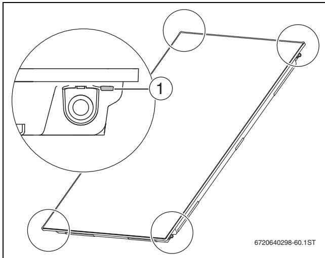
Bild 69 Belüftungsöffnungen
