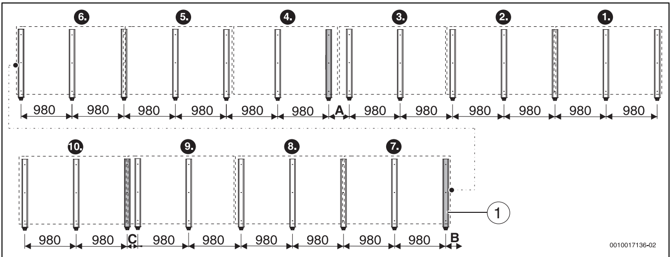
Bild 34 Grundausführung Beschwerungswannen, 10 waagerechte Kollektoren (Angaben in mm)
