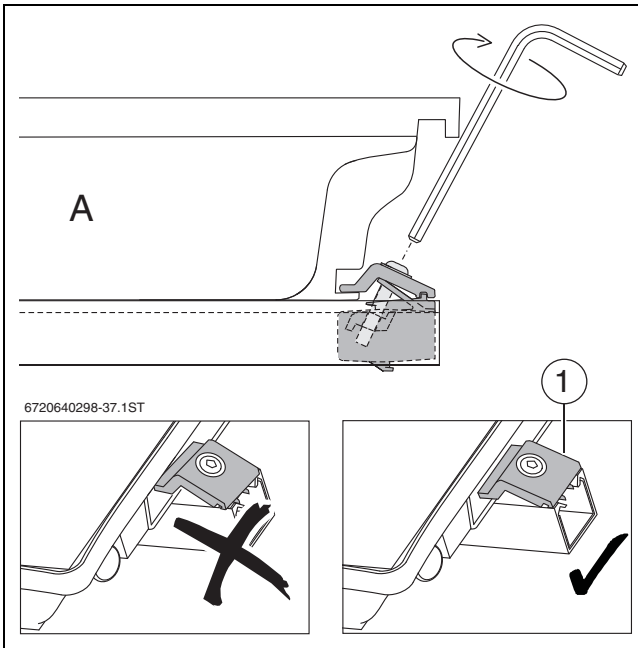
Bild 52 Kollektorspanner festdrehen
