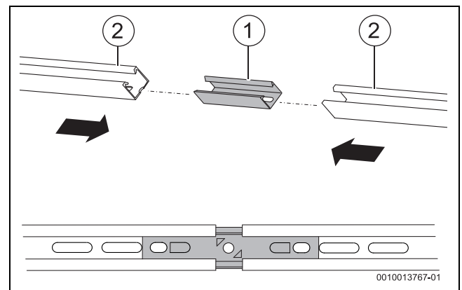
Bild 40 Profilschienen verbinden
