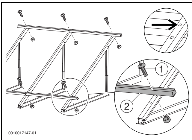
Bild 42 Profilschienen montieren
