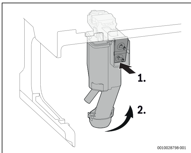
Bild 60 Kondensatsiphon herausnehmen
