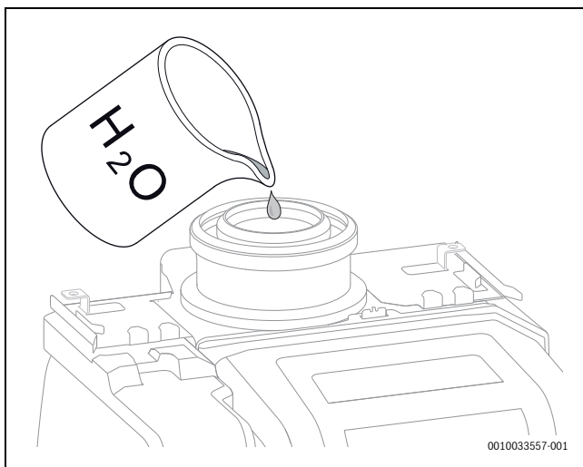
Bild 71 Kondensatsiphon mit Wasser füllen
