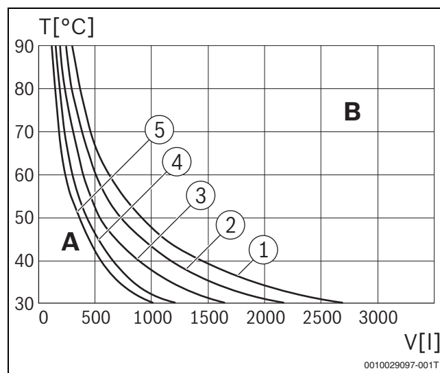
Bild 48 Kennlinien für Ausdehnungsgefäß (29 l)
