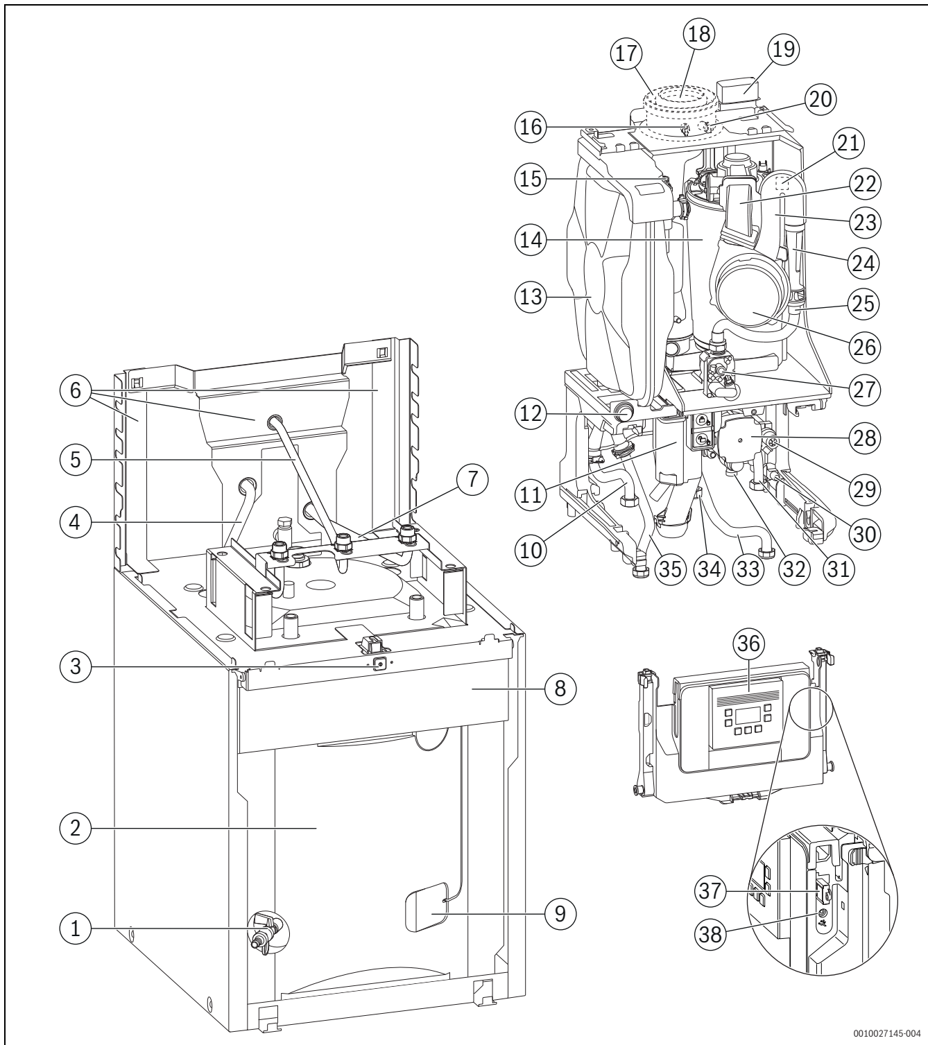
Bild 4 Produktübersicht
