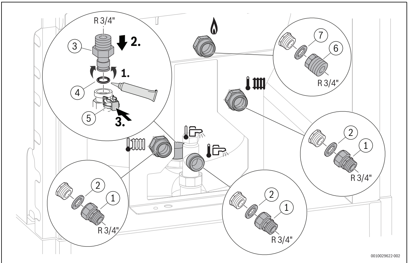
Bild 85 Zubehör CS 17 montieren
