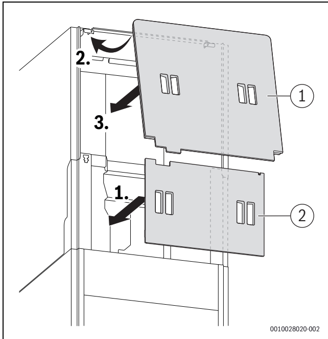
Bild 121 Wärmedämmung an der Rückseite anbringen (Zubehör SF 13)
