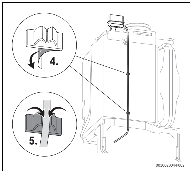
Bild 66 Kabelhalter an der Rückseite des Geräts anbringen und Kabel befestigen
