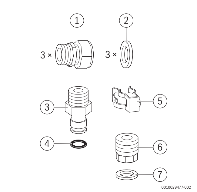
Bild 84 Lieferumfang Zubehör CS 17
