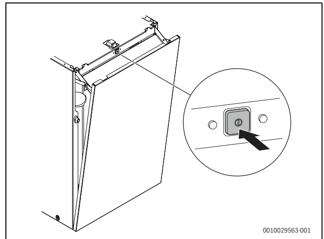
Bild 126 Gerät am Schalter Ein/Aus einschalten
