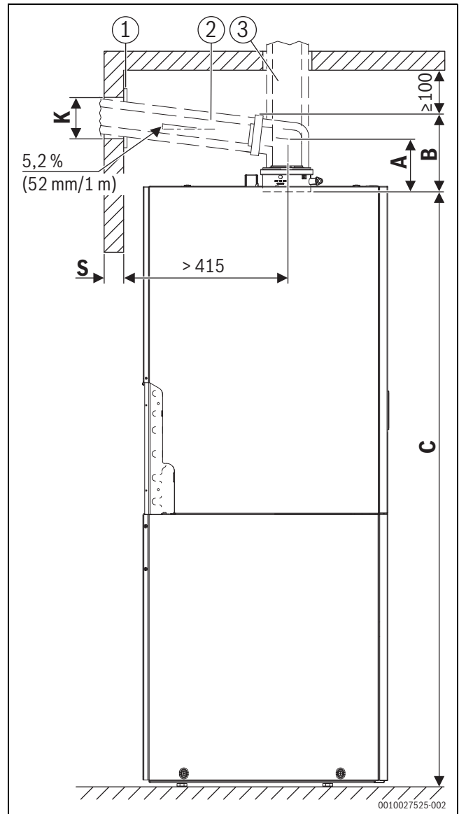
Bild 18 Ansicht von der linken Seite (Maße in mm)
