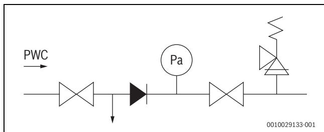
Bild 67 Beispiel: Sicherheitsgruppe für Expansionswasser nach EN 1488
