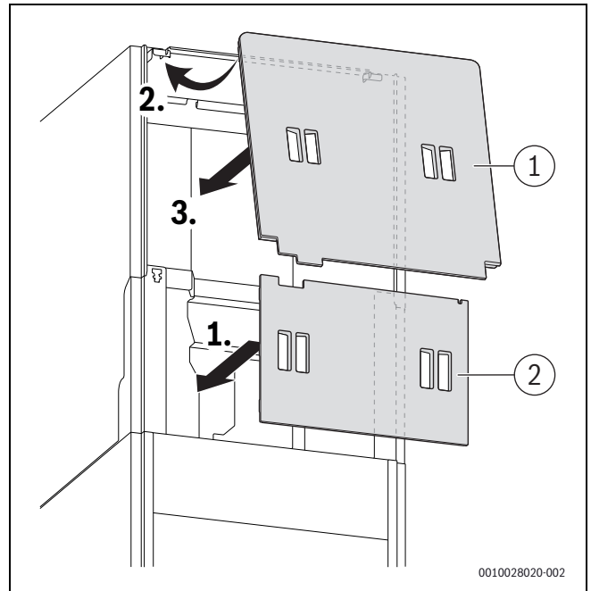
Bild 98 Zubehör SF 13 auf der Rückseite des Geräts anbringen
