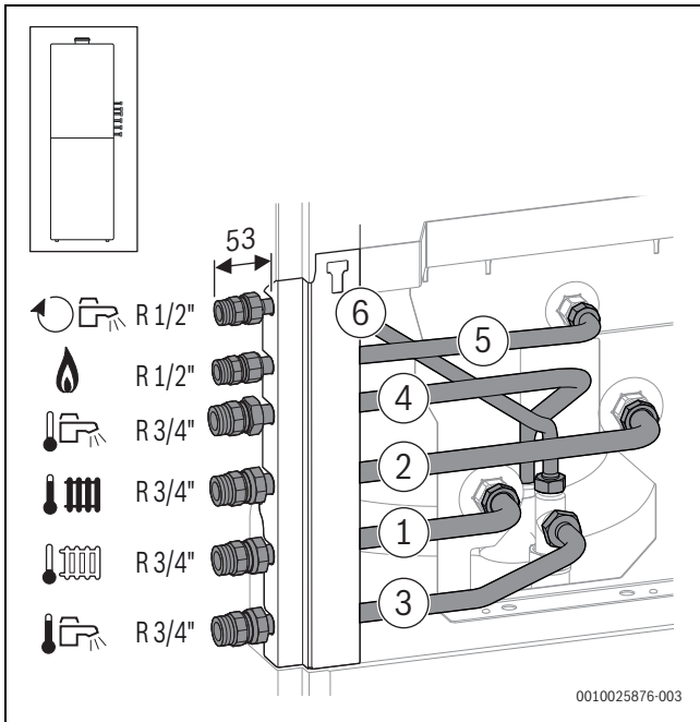
Bild 53 Zubehör CS 10 auf der rechten Seite montiert
