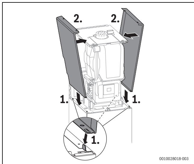
Bild 116 Seitenteile der Geräteverkleidung einsetzen
