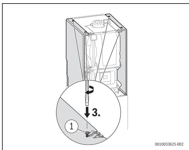
Bild 117 Seitenteile der Geräteverkleidung befestigen
