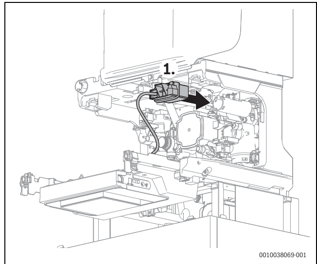
Bild 64 Funkmodul-Halter auf die Rückseite des Geräts führen
