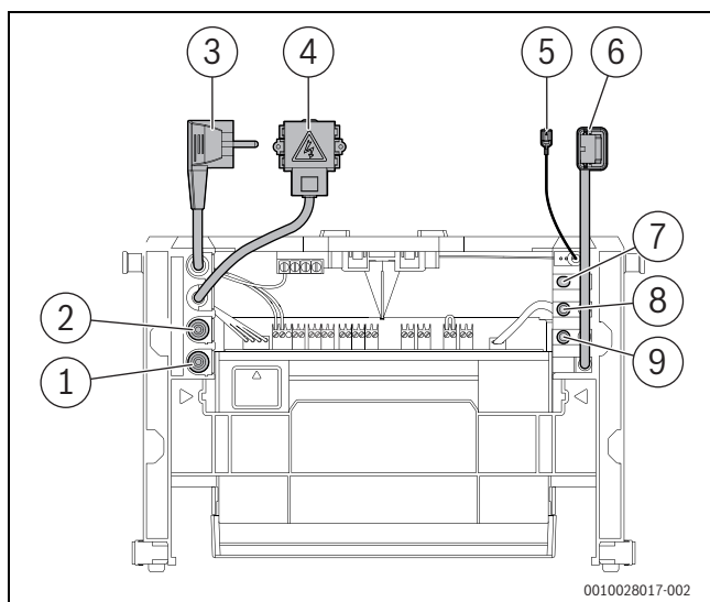
Bild 109 Lieferzustand des Steuergeräts mit angeschlossenen Komponenten
