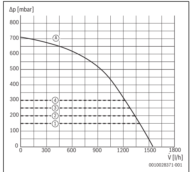
Bild 56 Pumpenkennfelder und Pumpenkennlinie (17/24 kW)
