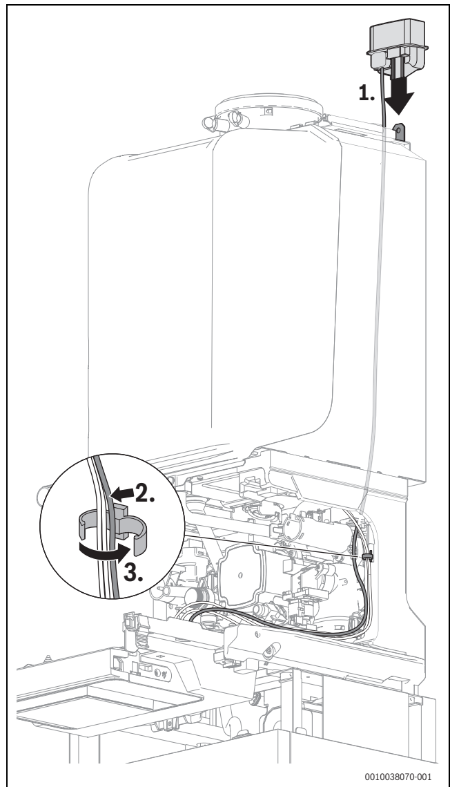
Bild 65 Funkmodul-Halter in den Steckplatz einsetzen und Kabel im Kabelhalter befestigen
