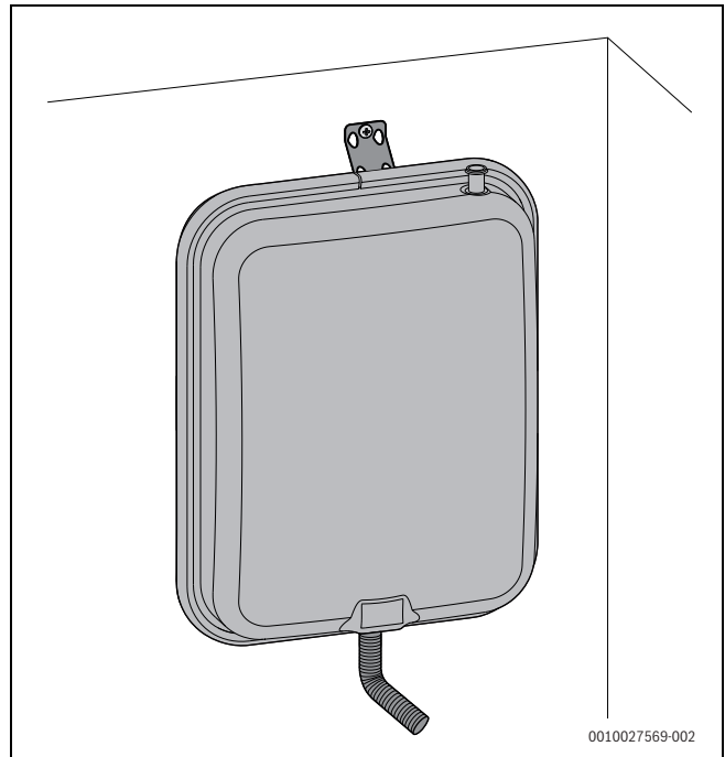
Bild 94 Zubehör EV 17 an der Wand montiert
