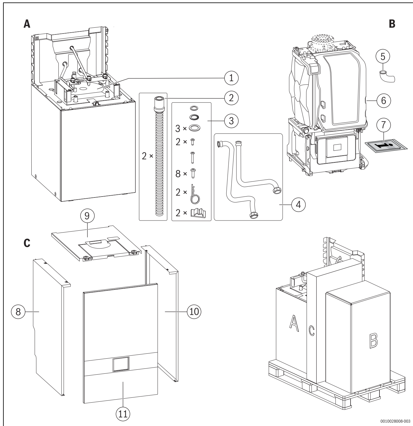
Bild 3 Lieferumfang
