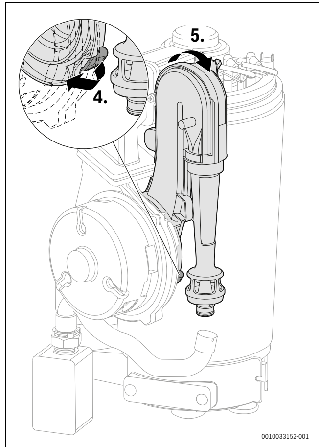
Bild 19 Venturirohr abnehmen
