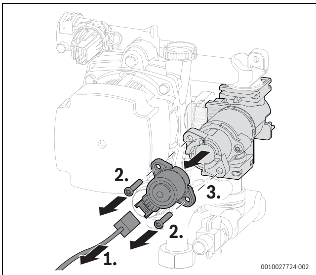
Bild 52 Motor am 3-Wege-Ventil ausbauen
