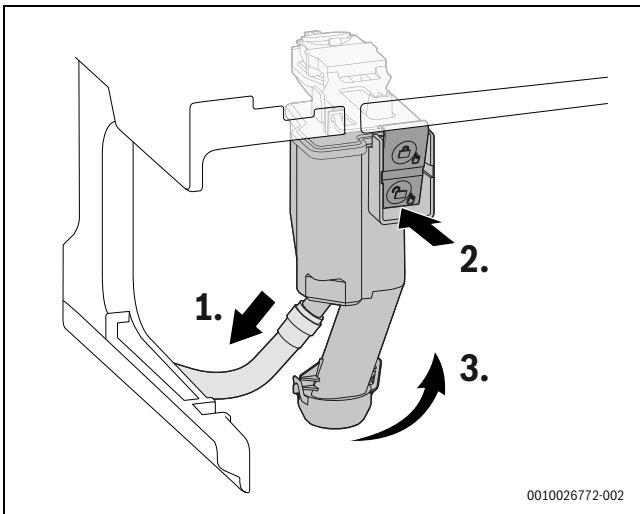
Bild 48 Kondensatsiphon ausbauen
