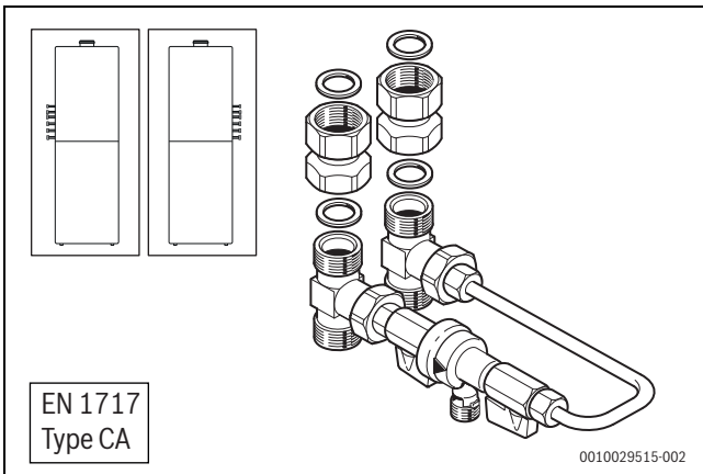
Bild 79 Lieferumfang Zubehör CS 30
