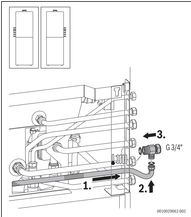
Bild 96 Anschluss des Zubehörs EV 17
