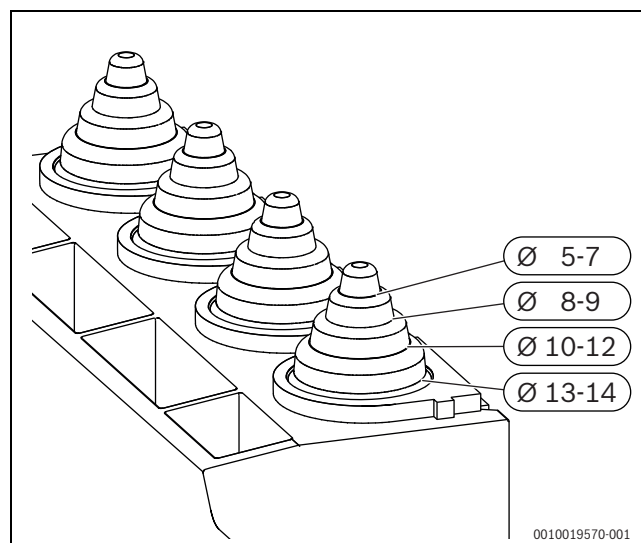
Bild 111 Zugentlastung an Kabeldurchmesser anpassen
