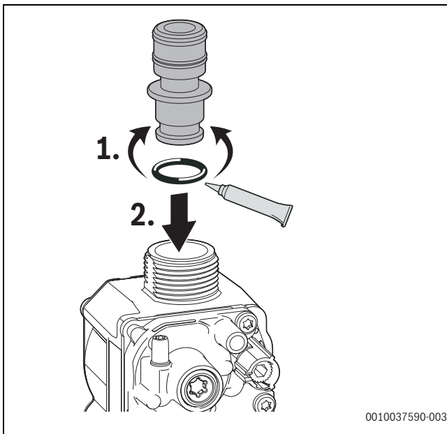
Bild 45 Gasdüse einsetzen
