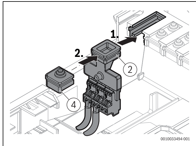
Bild 101 EMS-BUS-Leiste in die Öffnung für die Kabeldurchführungen einsetzen
