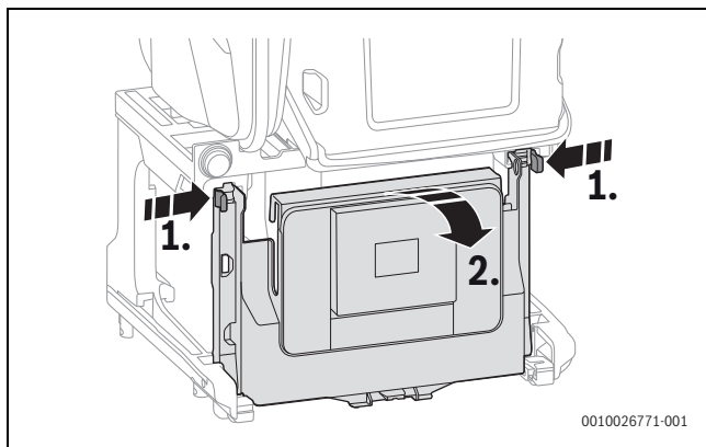
Bild 59 Steuergerät herunterklappen
