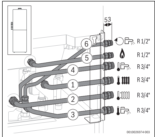
Bild 75 Zubehör CS 10 auf der linken Seite montiert
