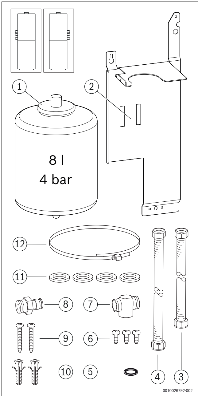
Bild 88 Lieferumfang Zubehör EVW 8
