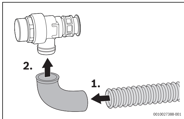
Bild 68 Schlauch am Sicherheitsventil anschließen
