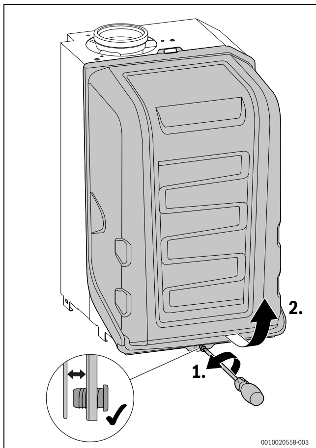
Bild 103 Brennerhaube abnehmen
