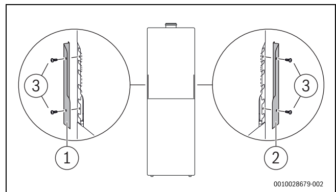
Bild 87 Zubehör SF 11 befestigen
