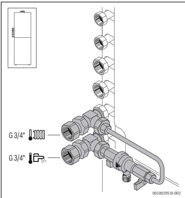
Bild 80 Zubehör CS 30 auf der linken Seite montiert
