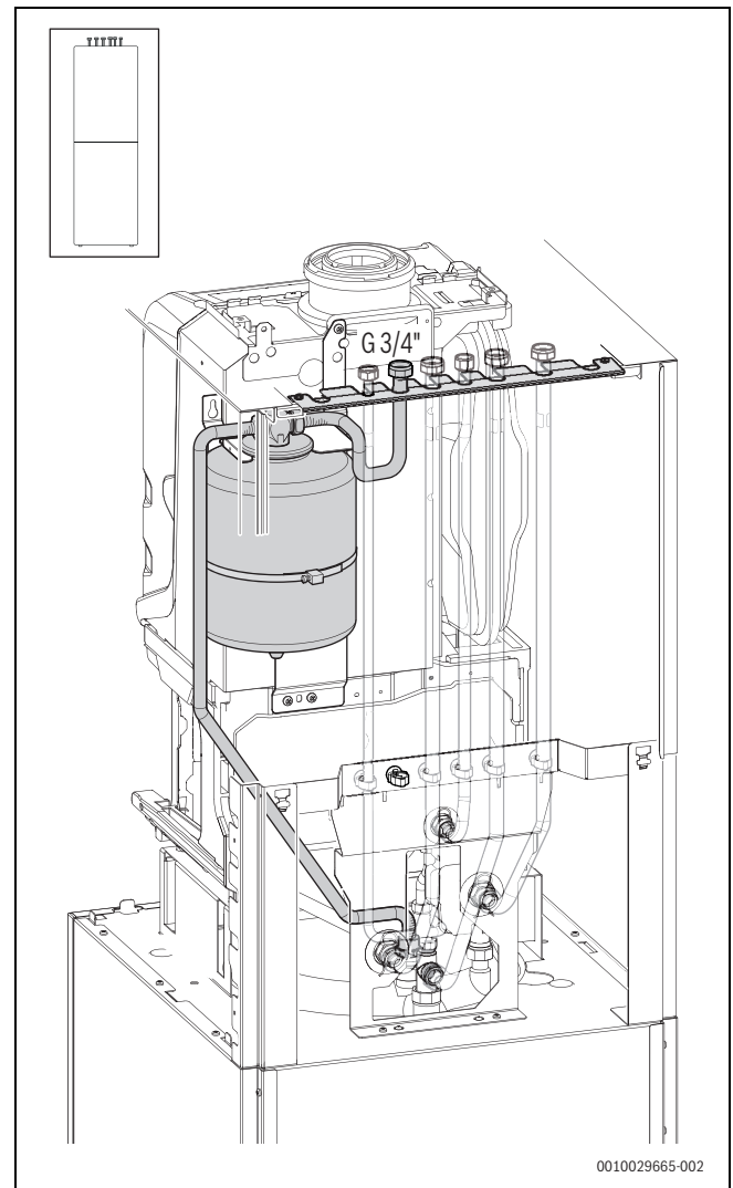
Bild 92 Zubehör EVW 8 im Gerät montiert mit vertikalem Anschluss-Set CS 33
