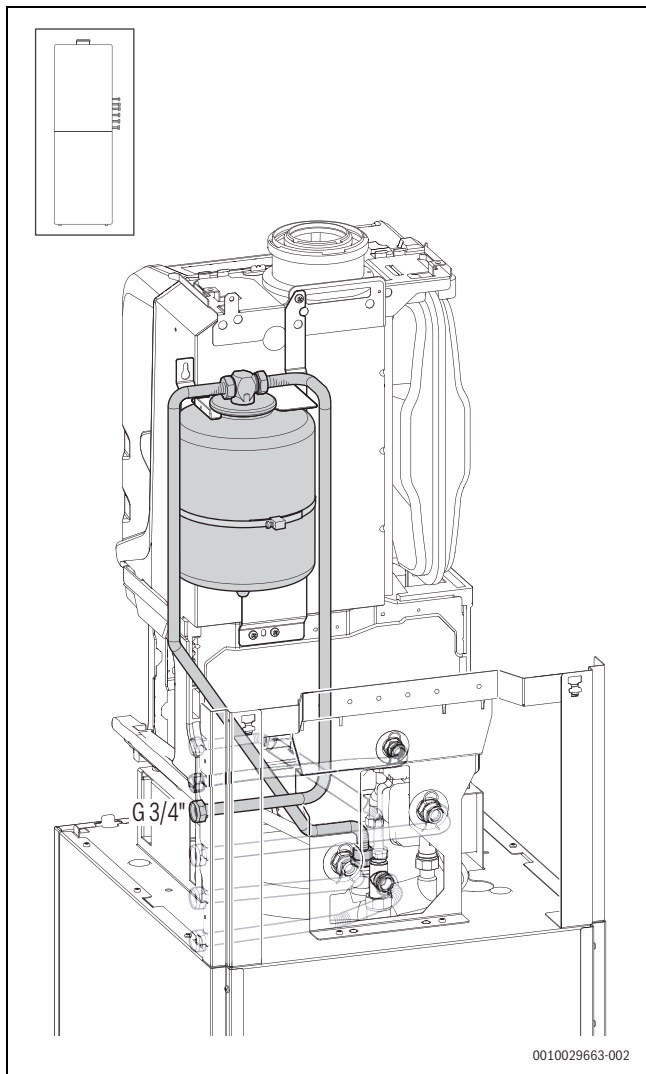
Bild 91 Zubehör EVW 8 im Gerät montiert mit horizontalem Anschluss-Set CS 10 auf der rechten Seite
