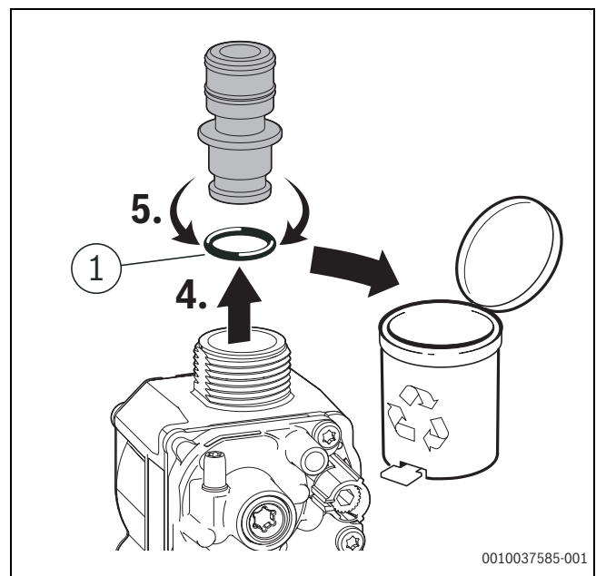
Bild 40 Gasdüse abnehmen
