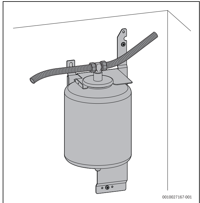
Bild 89 Zubehör EVW 8 an der Wand montiert
