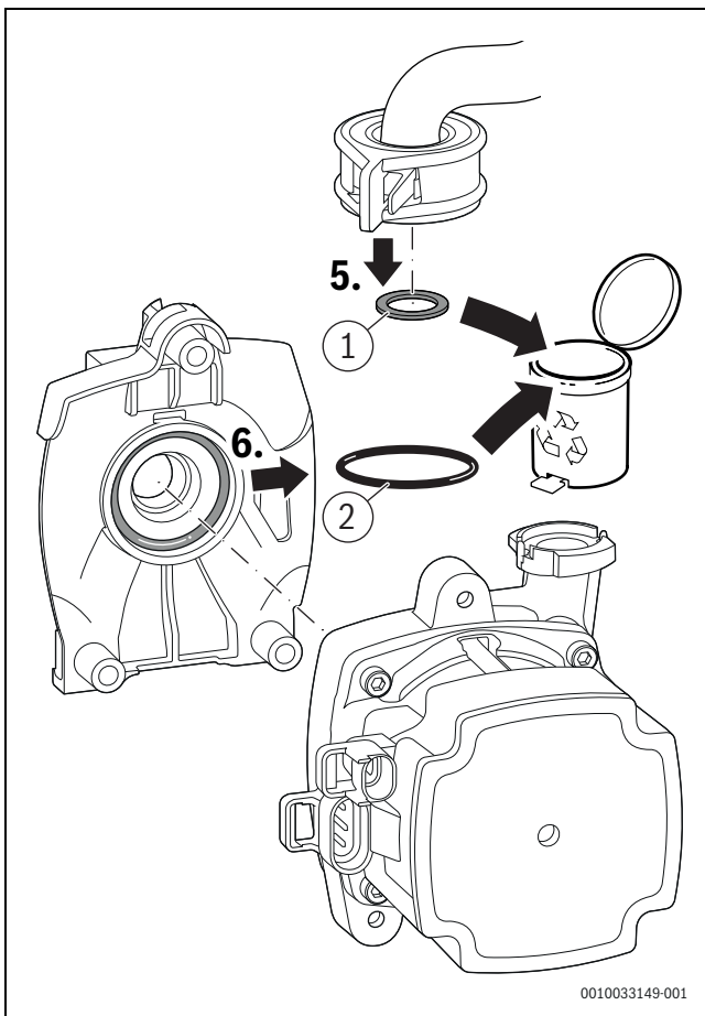
Bild 38 Dichtungen entsorgen
