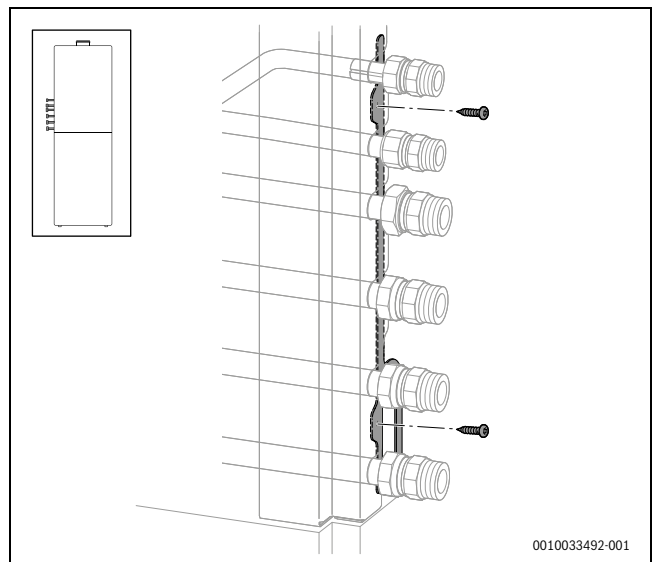
Bild 77 Abschluss der Montage auf der linken Seite
