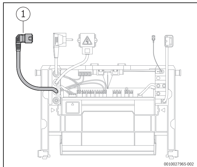
Bild 110 Steckplatz für das Anschlusskabel der Schichtladepumpe
