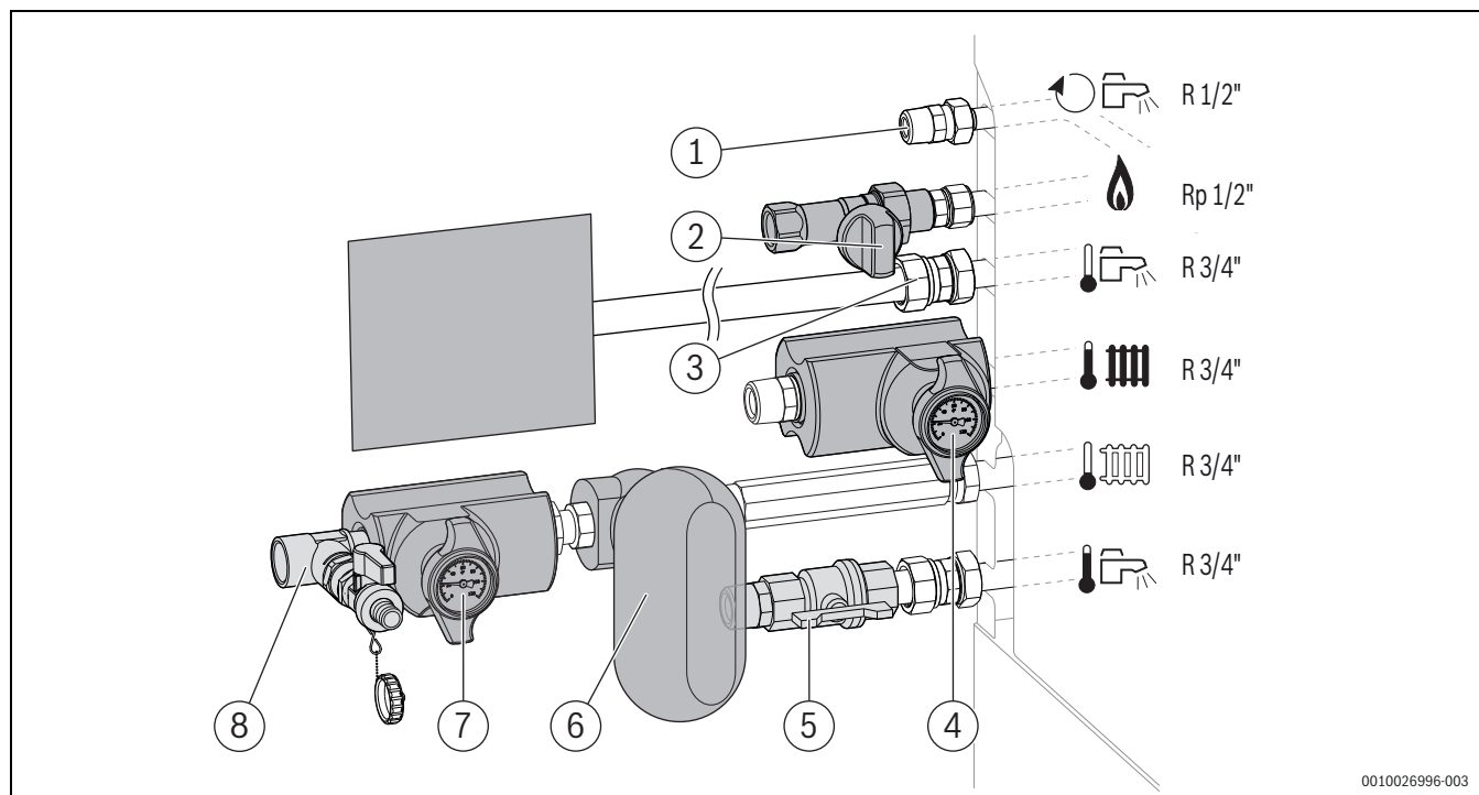
Bild 73 Armaturen-Set Zubehör CS 28-1 – Beispiel: Anschlüsse horizontal auf der linken Seite
