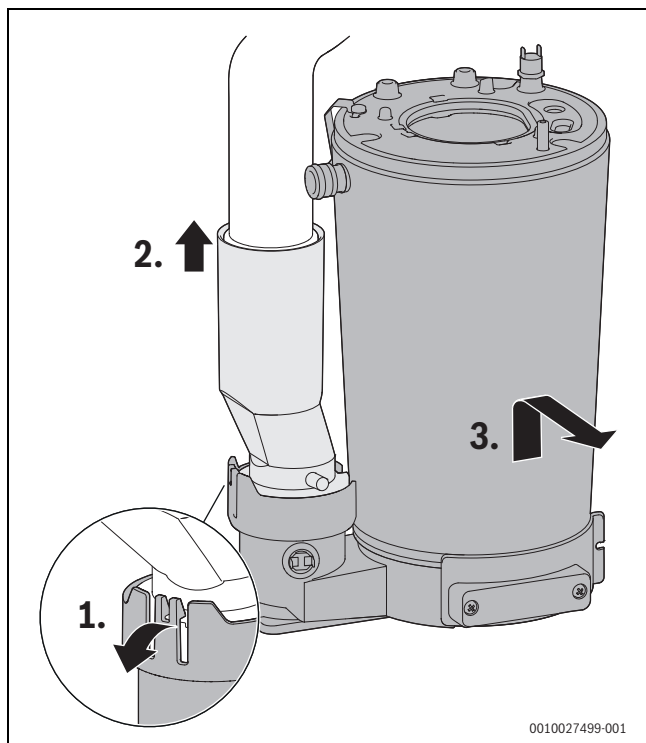
Bild 34 Wärmeblock ausbauen
