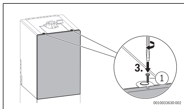
Bild 119 Vorderteil der Geräteverkleidung mit Schraube aus Lieferumfang sichern
