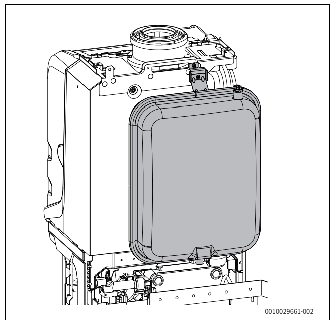
Bild 95 Zubehör EV 17 im Gerät montiert
