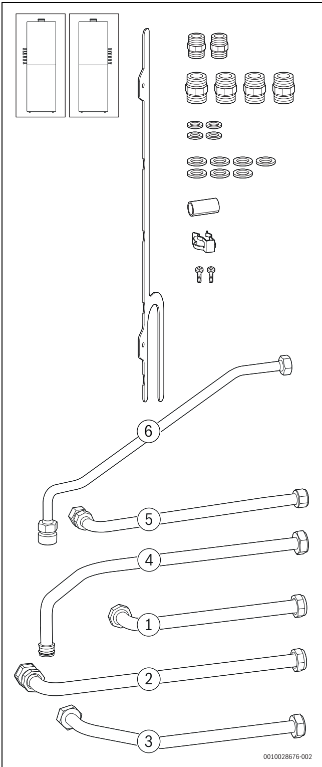
Bild 74 Lieferumfang Zubehör CS 10
