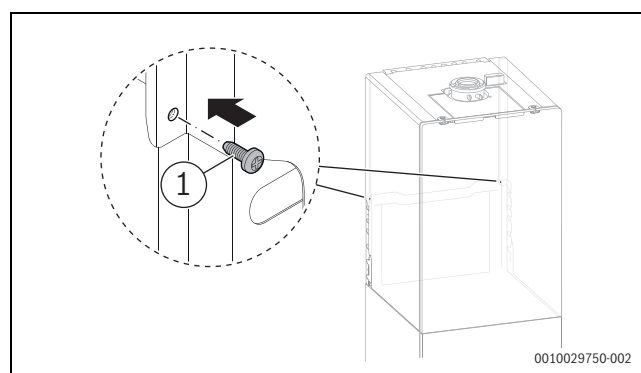
Bild 120 Seitenteile der Geräteverkleidung auf der linken und rechten Seite festschrauben
