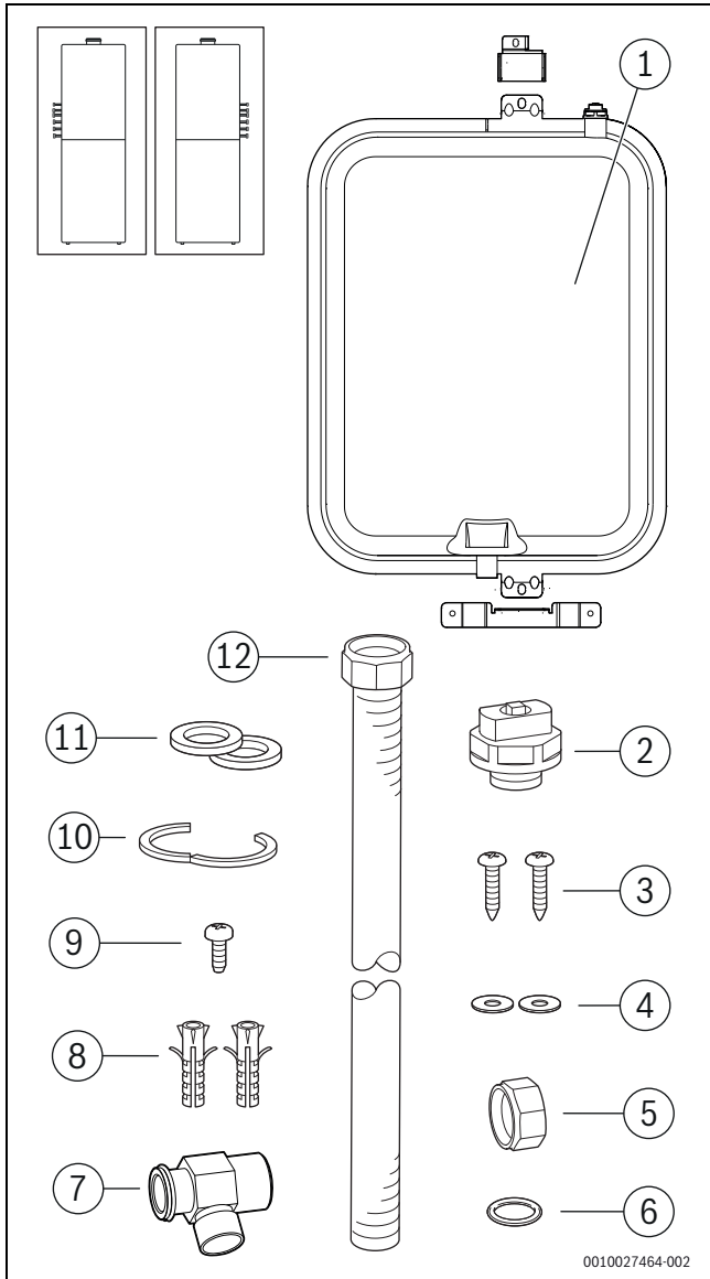
Bild 93 Lieferumfang Zubehör EV 17
