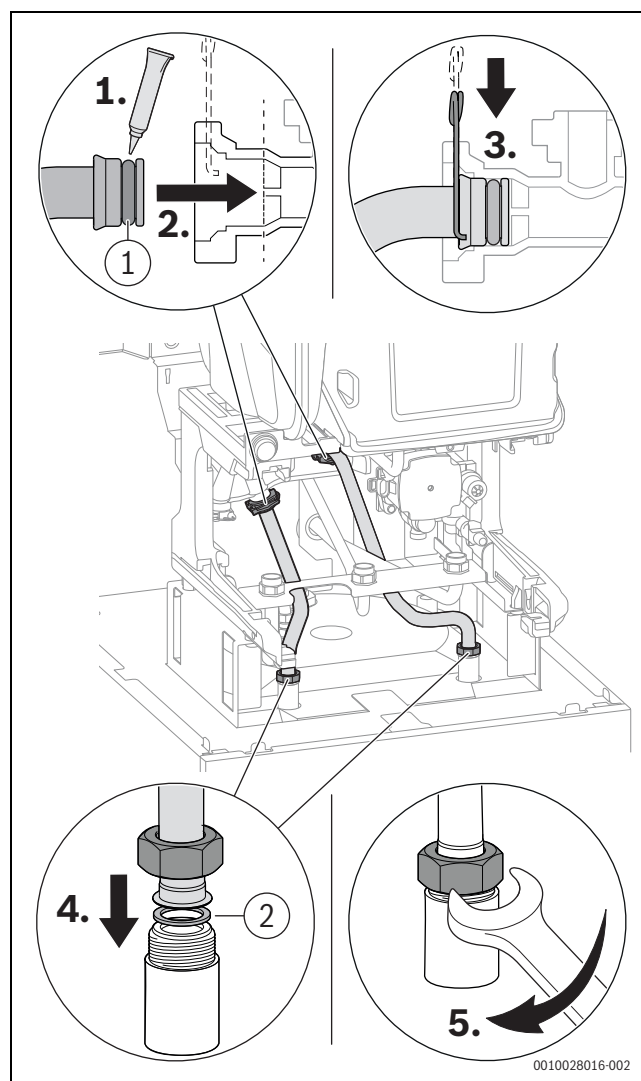
Bild 61 Vorlaufrohr und Rücklaufrohr zum Rohrwendelspeicher anschließen
