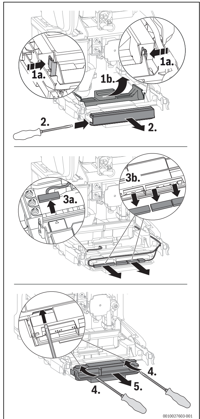
Bild 47 Steuergerät herausnehmen
