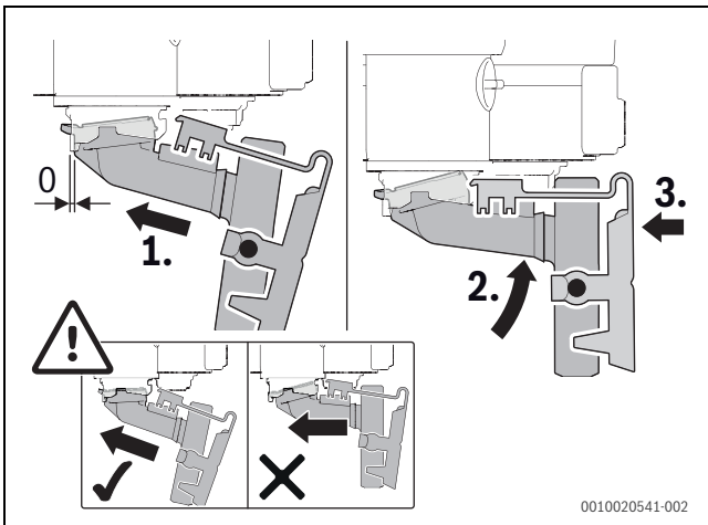
Bild 63 Kondensatsiphon wieder einsetzen und auf festen Sitz prüfen
