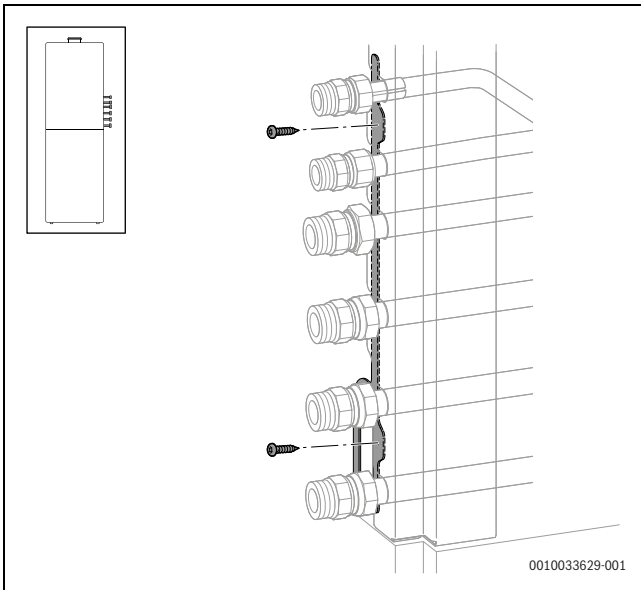
Bild 78 Abschluss der Montage auf der rechten Seite
