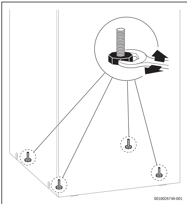
Bild 122 Am endgültigen Aufstellort Unebenheiten des Fußbodens mit den Stellfüßen ausgleichen
