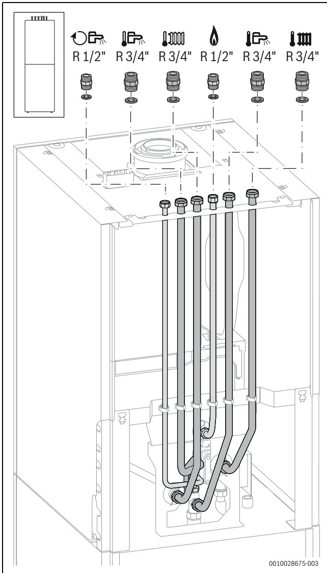
Bild 54 Zubehör CS 33 montiert
