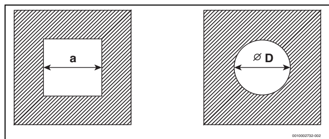
Bild 19 Quadratischer und runder Querschnitt
