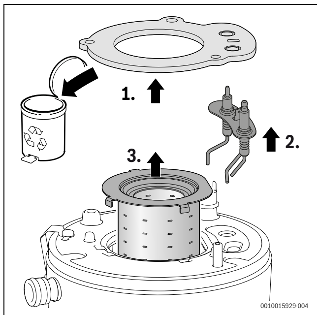
Bild 24 Brenner herausnehmen
