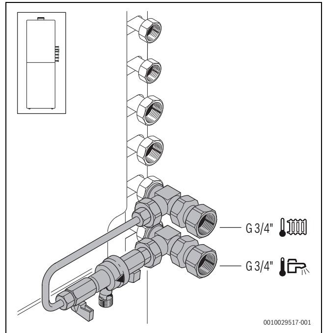
Bild 81 Zubehör CS 30 auf der rechten Seite montiert
