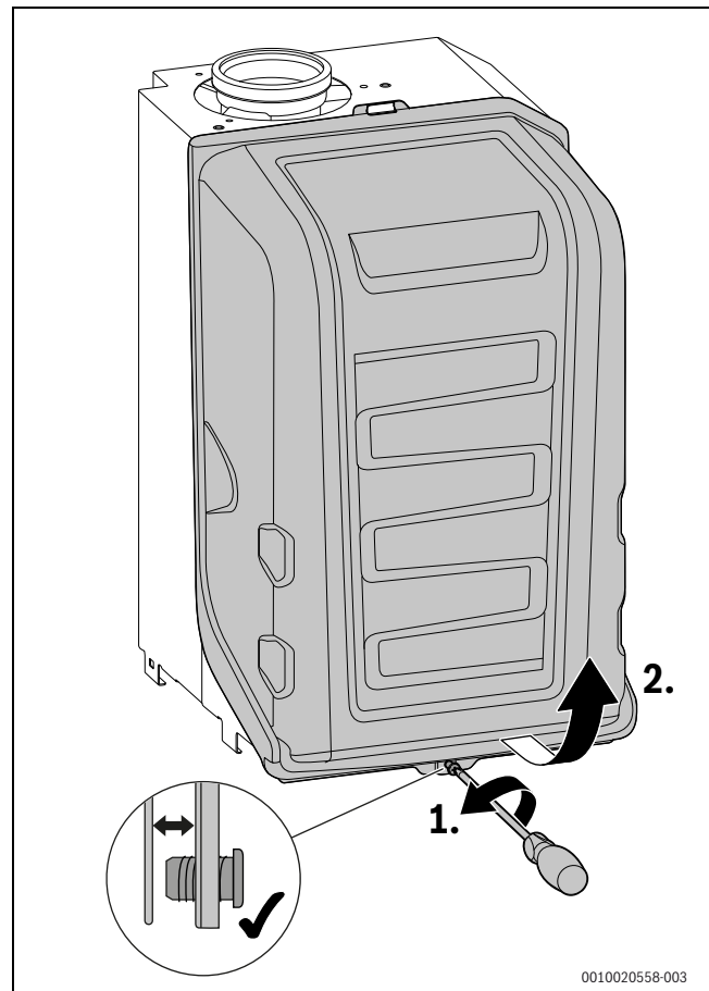
Bild 3 Brennerhaube abnehmen
