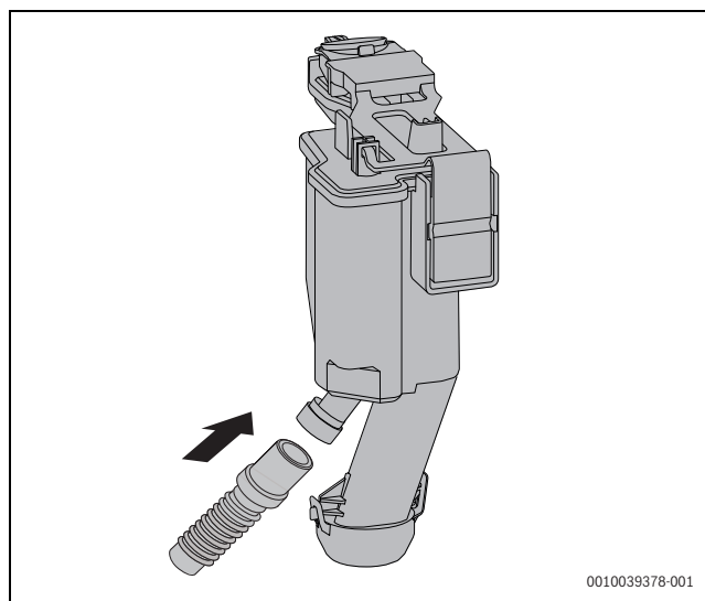
Bild 69 Schlauch am Kondensatsiphon anschließen
