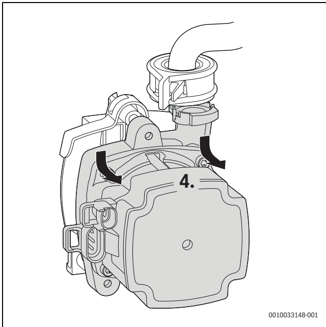
Bild 37 Heizungspumpe abnehmen
