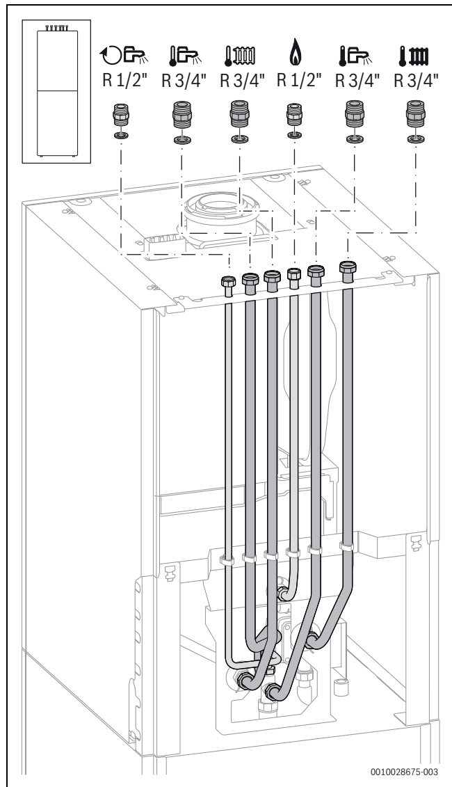
Bild 83 Zubehör CS 33 montiert
