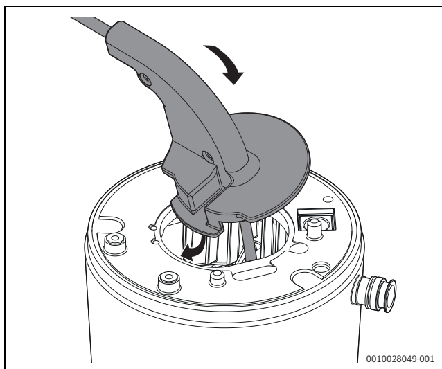
Bild 27 Bürste in den Wärmeblock einsetzen
