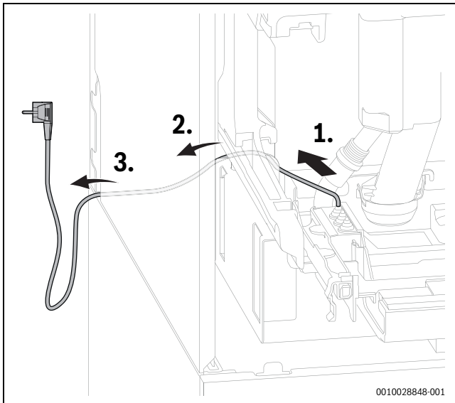
Bild 114 Kabelführung des Netzkabels
