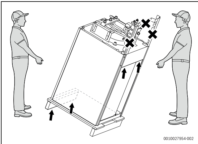
Bild 49 Transport des Speichers
