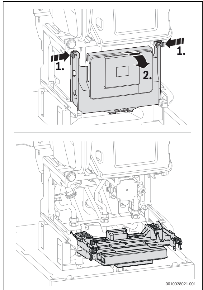
Bild 15 Steuergerät herunterklappen
