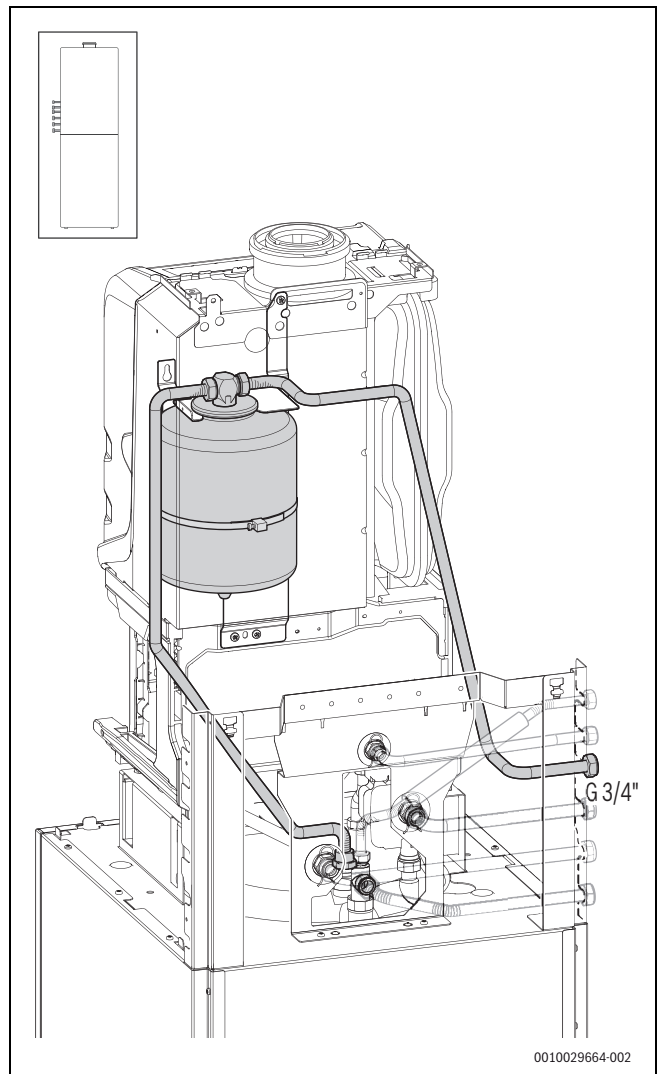
Bild 90 Zubehör EVW 8 im Gerät montiert mit horizontalem Anschluss-Set CS 10 auf der linken Seite
