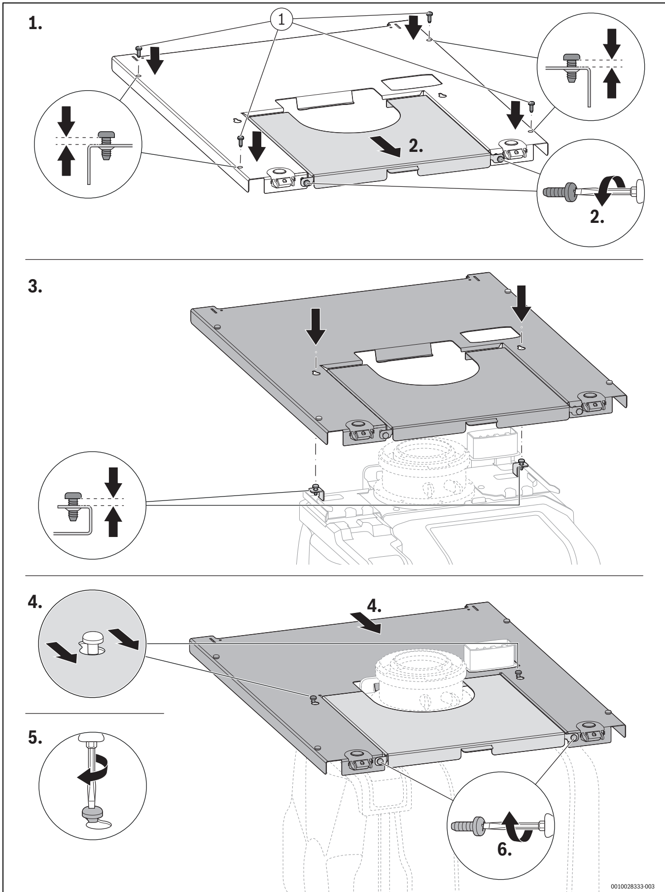
Bild 115 Oberteile der Geräteverkleidung befestigen. Wenn erforderlich können beide Teile der Verkleidung nacheinander eingesetzt werden.
