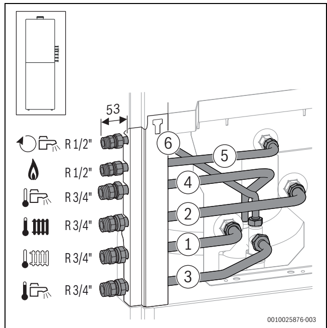
Bild 76 Zubehör CS 10 auf der rechten Seite montiert
