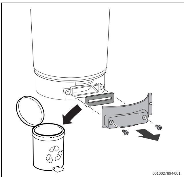
Bild 30 Prüföffnung öffnen
