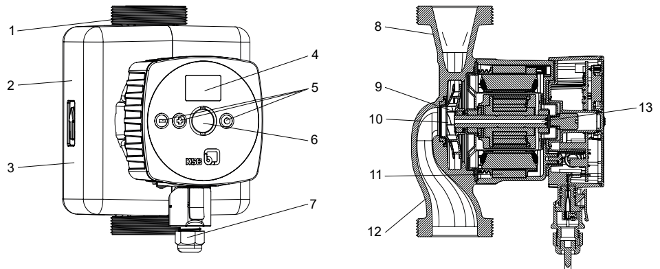
Abb. 2: Darstellung Pumpenaggregat
