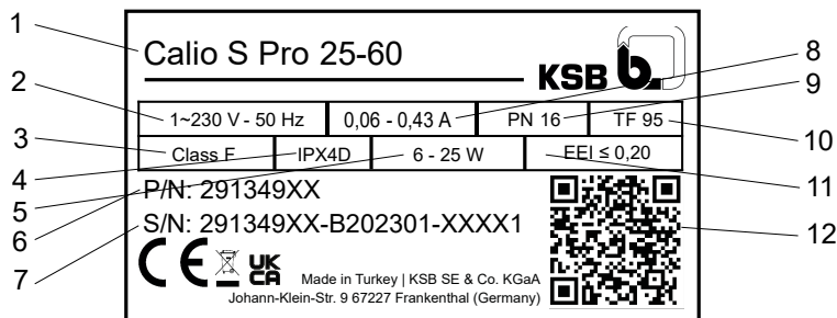
Abb. 1: Typenschild (Beispiel)
