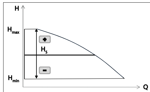
Abb. 10: Einstellung Konstantdruckregelung
