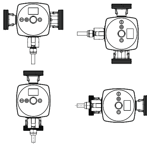
Abb. 3: Zulässige Einbaulagen
