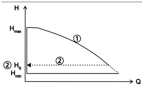
Abb. 9: Funktion Konstantdruckregelung
