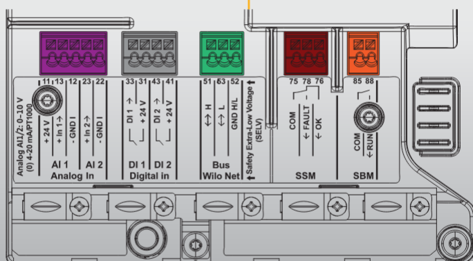
Anschlussklemmen
