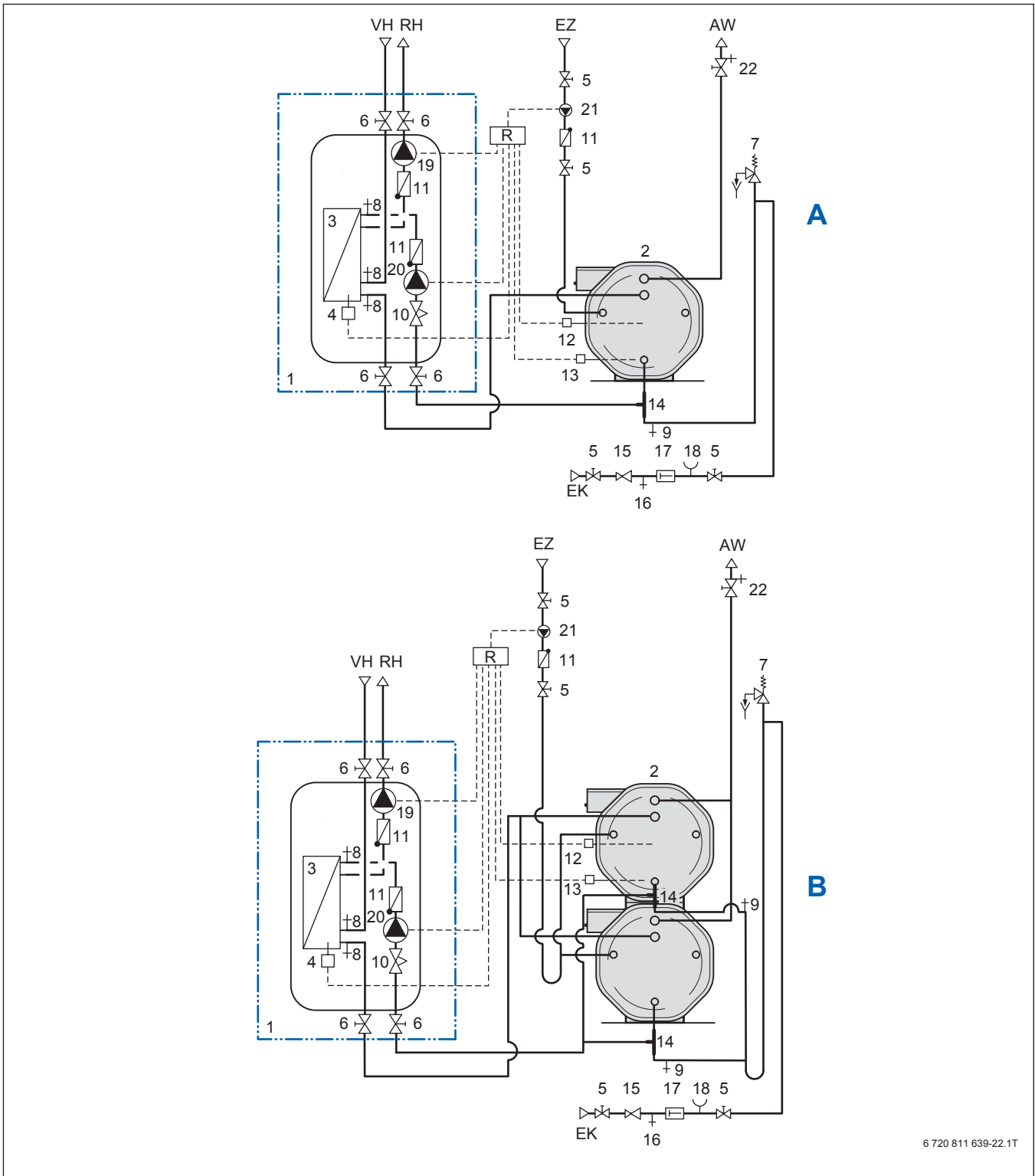
Bild 127 Hydraulischer Anschluss Wärmetauscher-Set Logalux SLP in Verbindung mit einem bzw. 2 Warmwasserspeichern Logalux LF im Speicherladesystem; Prinzipbild gilt grundsätzlich auch für stehende Warmwasserspeicher Logalux SF (→ Bild 125, Seite 143 und Bild 126, Seite 144)
