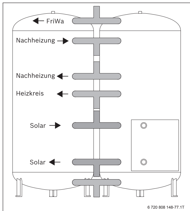
Bild 173 2 Logalux PNR.../5 mit Kaskadierungssets mit T-Stück
