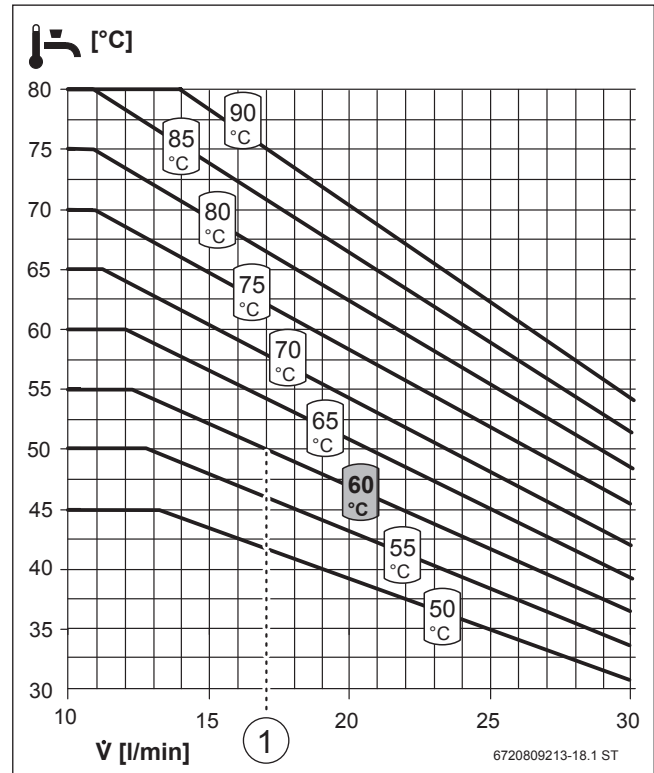
Bild 135 Temperaturverhalten Frischwasserstation
