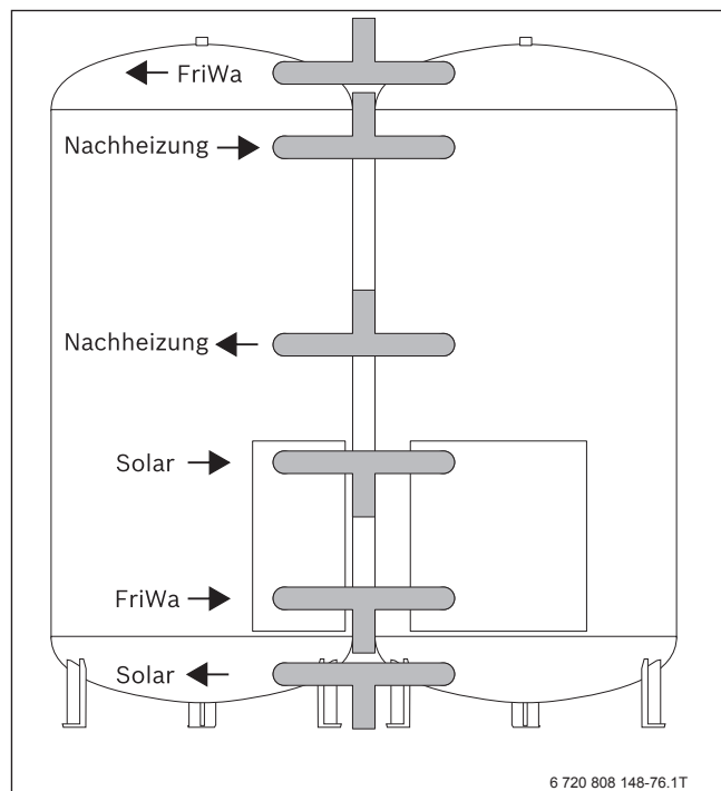
Bild 172 2 Logalux PR.../5 E mit Kaskadierungssets mit R 1 1/2 T-Stück
