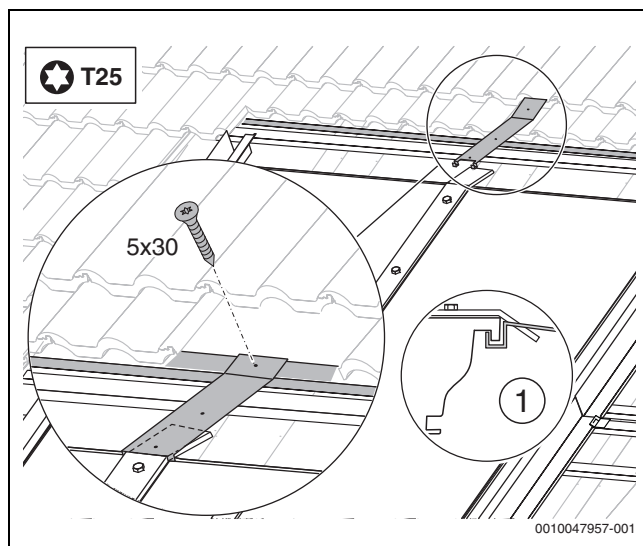
Bild 66 Senkrechte Ausführung
