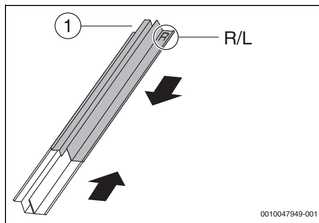
Bild 58 Seitliche Eindeckbleche ineinanderschieben (senkrecht)
