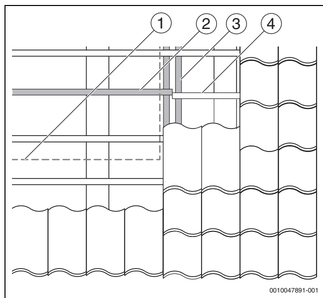
Bild 23 Dachlatte versetzen
