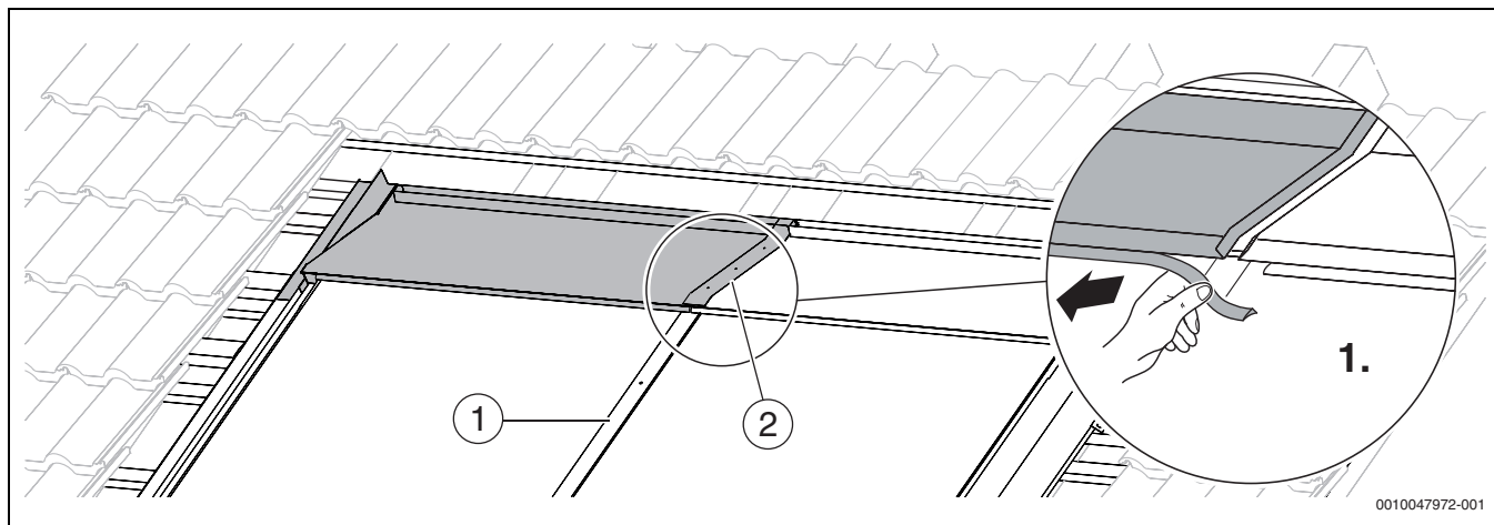
Bild 81 Dichtlippe abziehen
