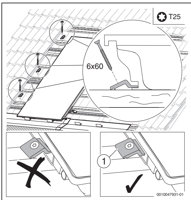
Bild 40 Niederhalter festschrauben
