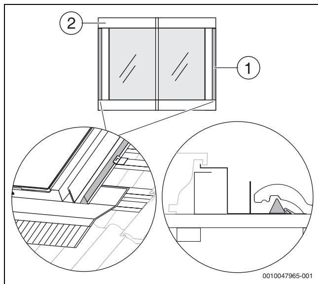
Bild 73 Dreieckdichtband einlegen
