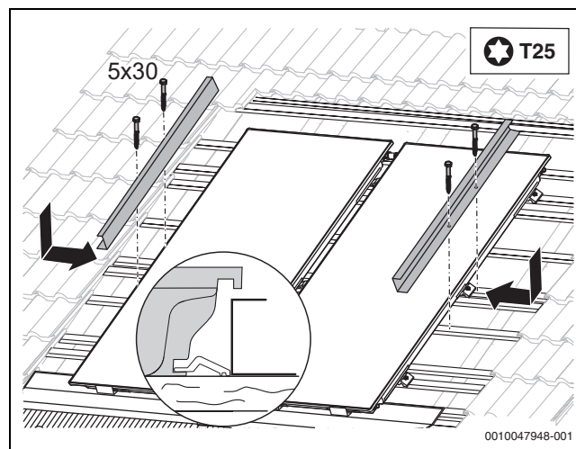
Bild 57 Seitliche Stützbleche montieren
