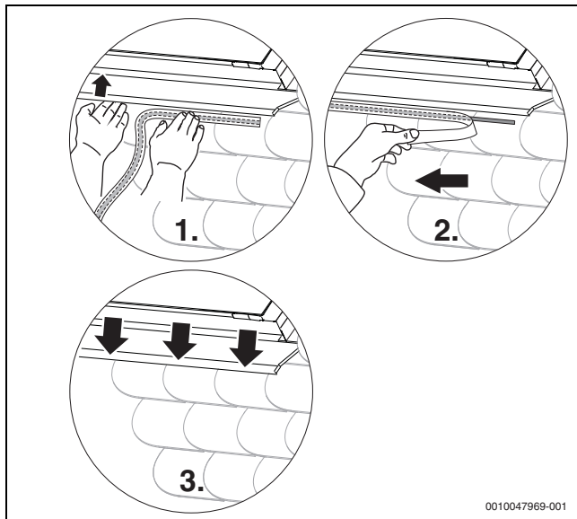
Bild 77 Unteres Eindeckblech auf Eindeckung kleben
