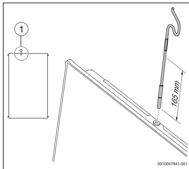
Bild 51 Kollektorfühler montieren
