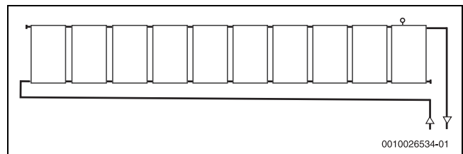
Bild 13 Wechselseitiger Anschluss 1 Reihe
