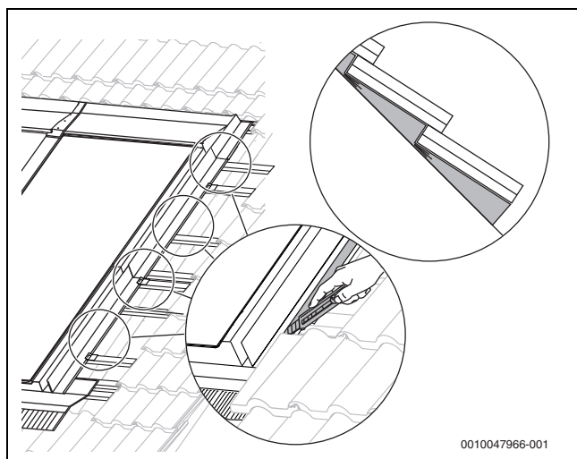
Bild 74 Dreieckdichtband einschneiden
