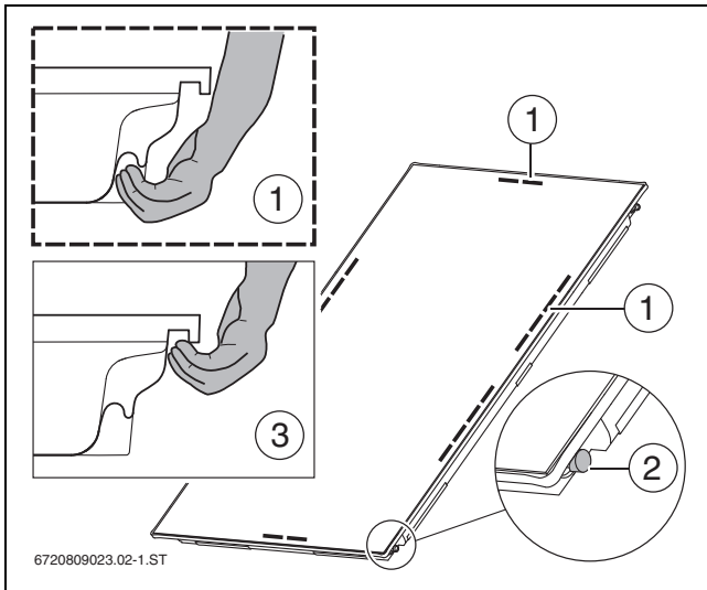
Bild 16 Kollektor tragen
