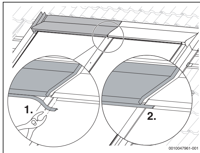
Bild 70 Dichtlippe anpassen
