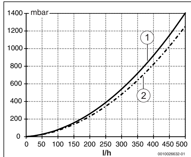
Bild 3 Druckverlustkurve (Wasser-Glykol-Gemisch)
