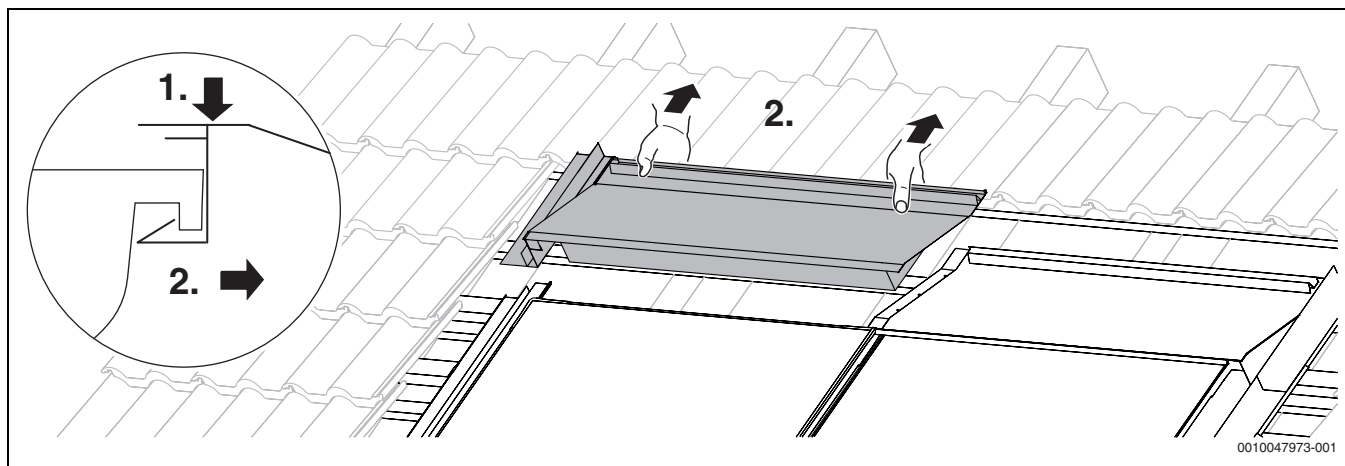
Bild 82 Eindeckblech abziehen
