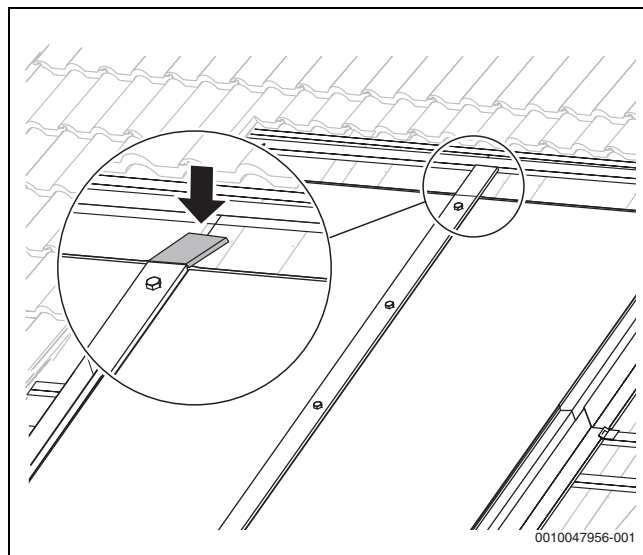
Bild 65 Oberes Ende leicht nach unten drücken
