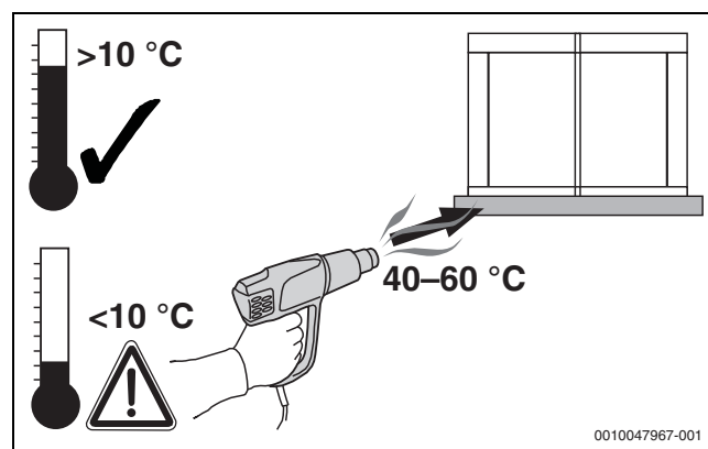
Bild 75 Bleischürze erwärmen, wenn erforderlich
