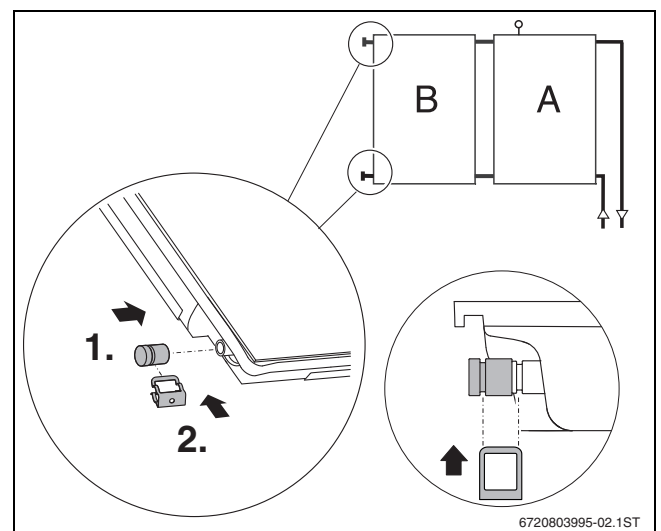
Bild 34 Kappen montieren
