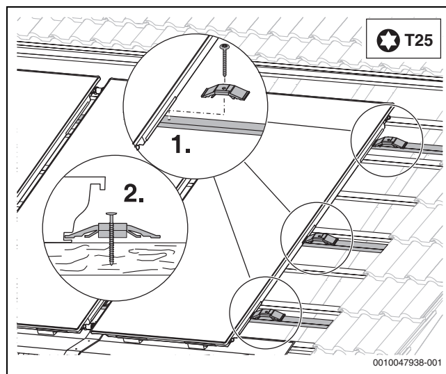
Bild 48 Weitere Niederhalter montieren
