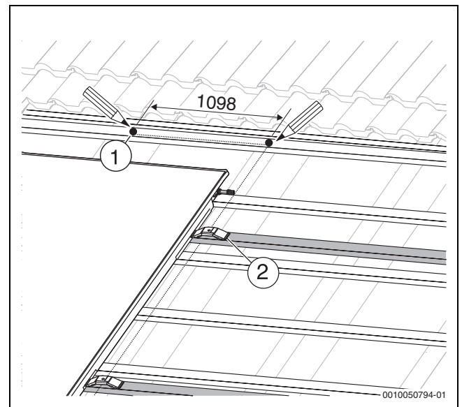
Bild 42 Montageposition des oberen Verbinders bei waagerechten Kollektoren
