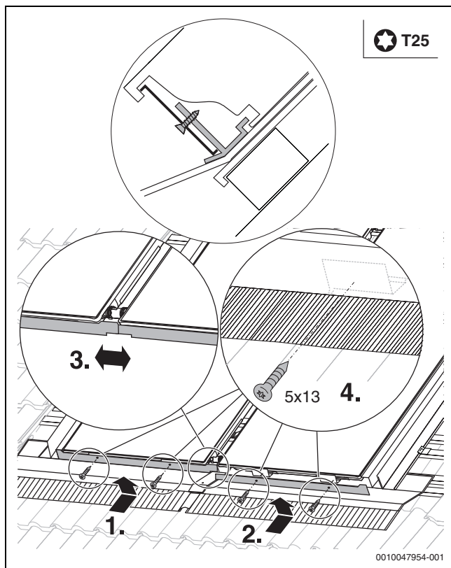
Bild 63 Blenden festschrauben
