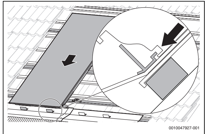
Bild 37 Linken Kollektor auflegen
