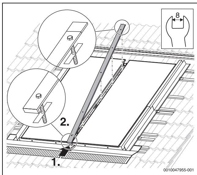
Bild 64 Abdeckleiste montieren
