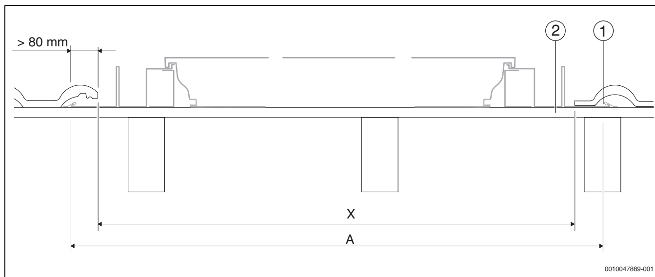
Bild 21 Kollektorfeldbreite
