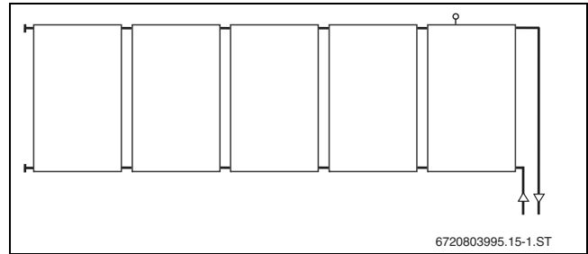
Bild 12 Gleichseitiger Anschluss rechts oder links (1 Reihe)
