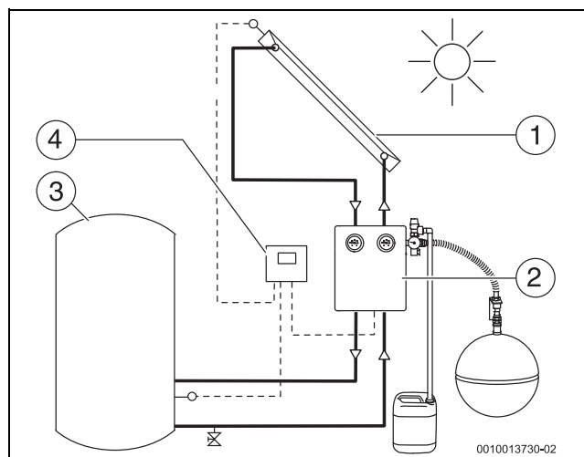
Bild 9 Beispielhafte Darstellung einer Solaranlage
