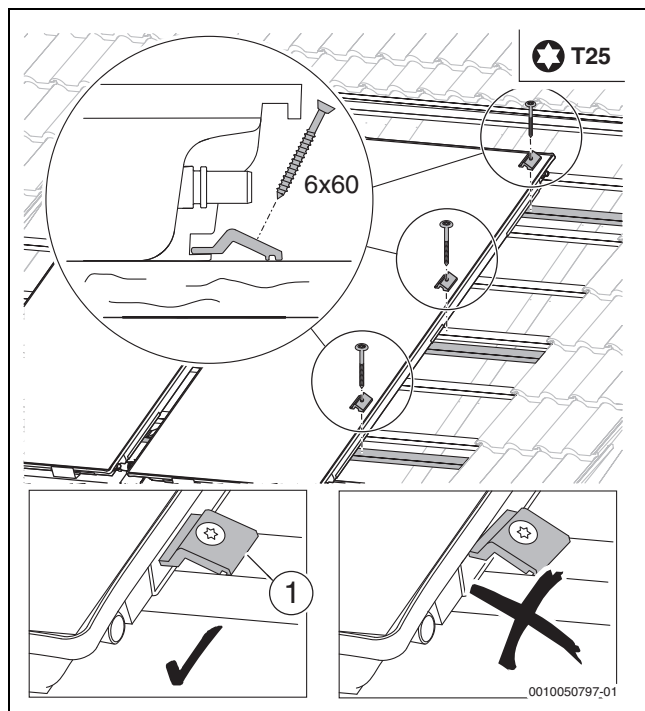
Bild 49 Niederhalter festschrauben
