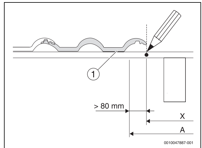
Bild 19 Maß X
