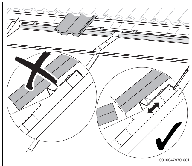
Bild 78 Dachziegelaufgabe positionieren
