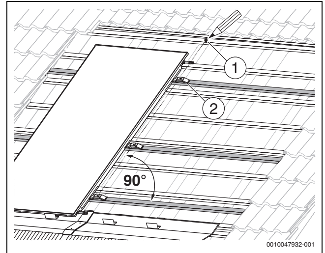
Bild 41 Montageposition des oberen Verbinders
