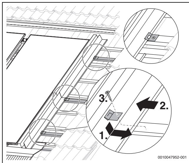
Bild 61 Hafter montieren
