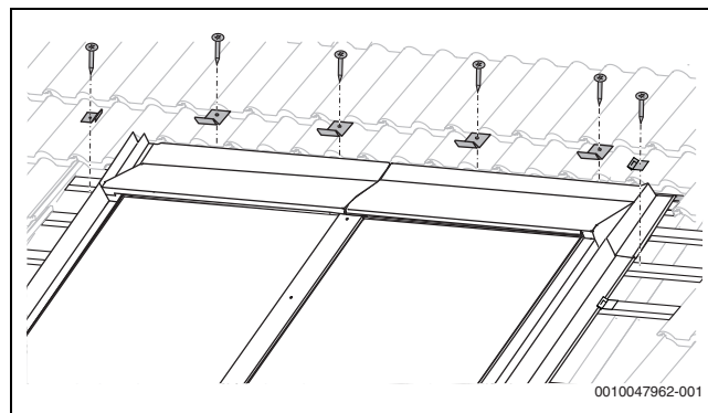
Bild 71 Obere Eindeckbleche mit Haftern fixieren
