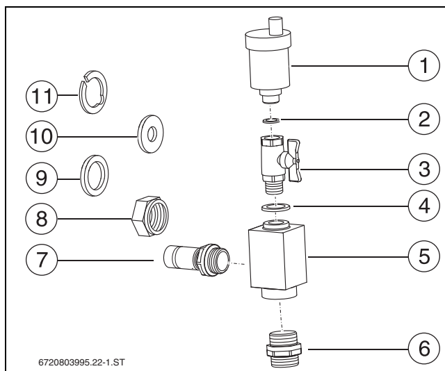
Bild 55 Lieferumfang Entlüfter-Set
