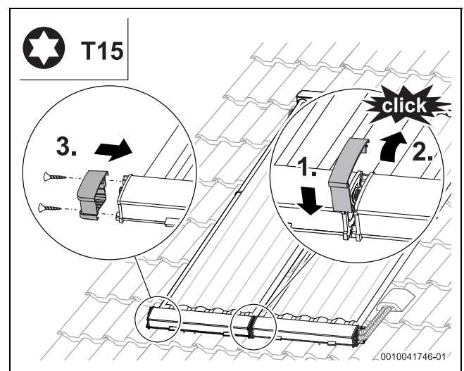
Bild 60 Endkappen montieren (hier: gleichseitiger Anschluss)
