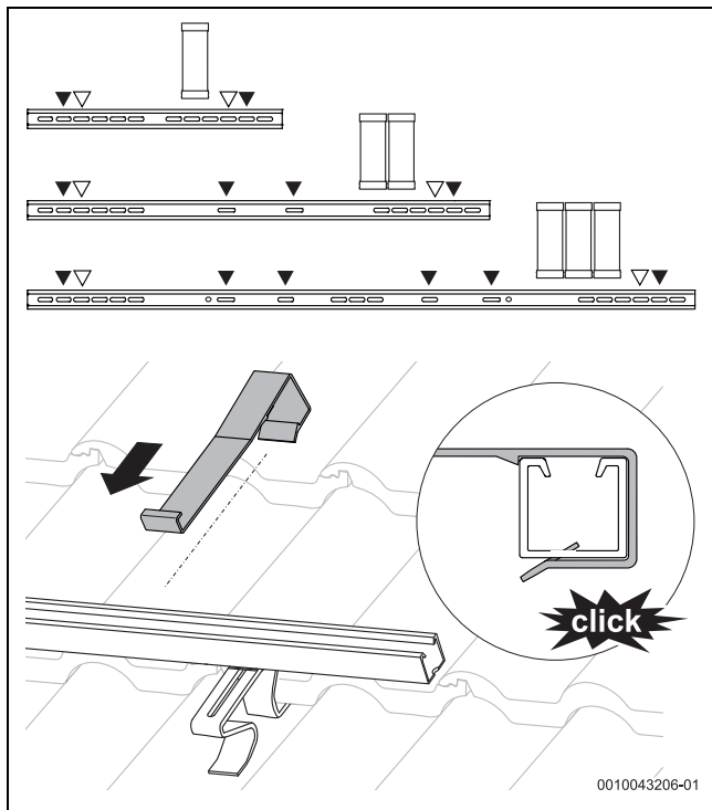
Bild 41 Abrutschsicherung montieren
