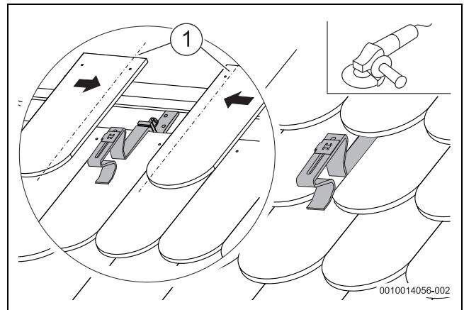
Bild 28 Biberschwanzziegel anpassen
