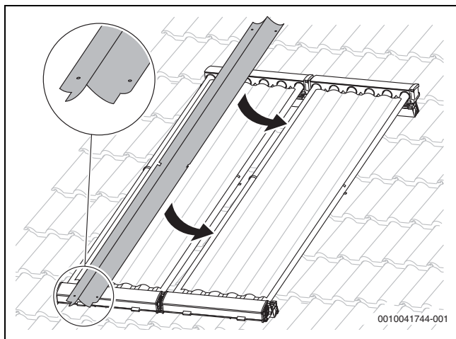
Bild 58 Zwischenspiegel einlegen
