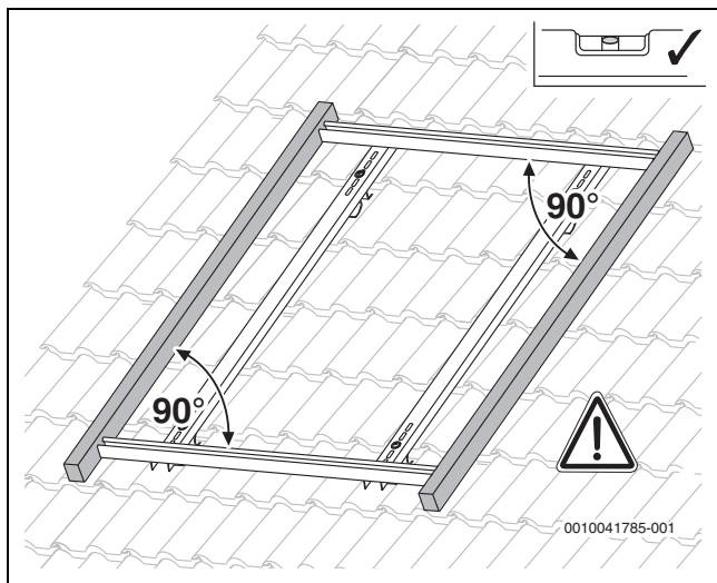
Bild 40 Profilschienen ausrichten
