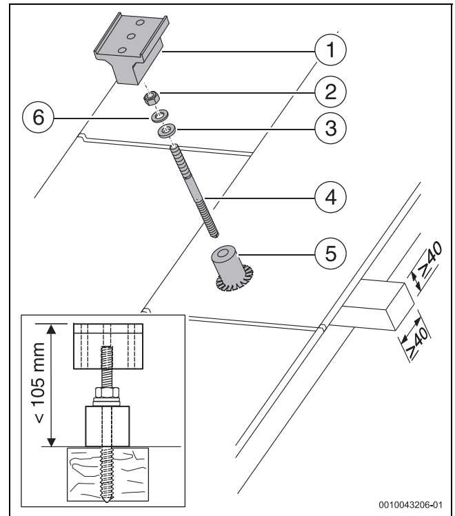
Bild 30 Stockschraube montieren
