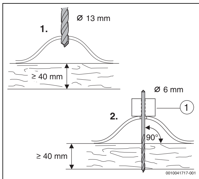
Bild 32 Vorbohren
