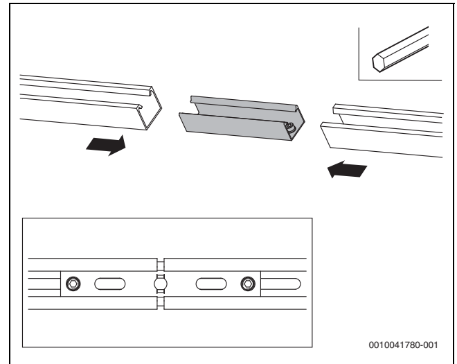
Bild 38 Profilschienen verbinden
