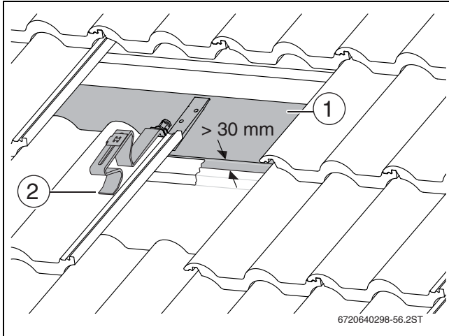
Bild 25 Sparrenanker auf Brett/Bohle montieren
