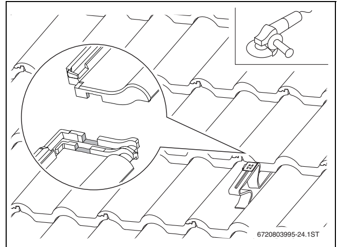
Bild 23 Dachziegel anpassen
