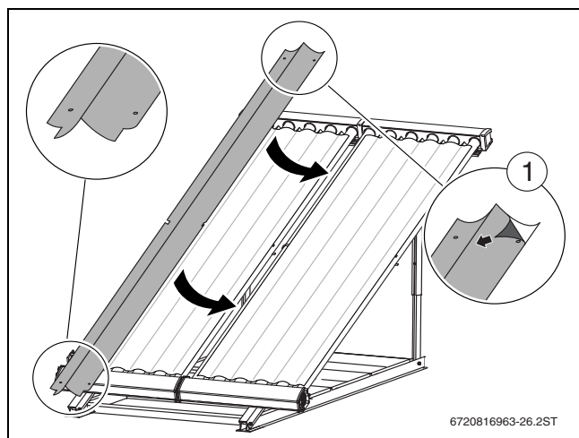
Bild 58 Zwischenspiegel einlegen
