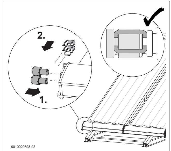
Bild 56 Entlüfterstopfen montieren (hier: gleichseitiger Anschluss)
