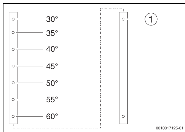
Bild 25 Neigungswinkel über Löcher in der Schiene wählen
