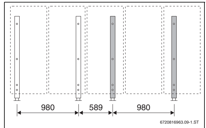
Bild 30 Grundausführung für 2 Kollektoren und Erweiterung für 3 Kollektoren (Maße in mm)
