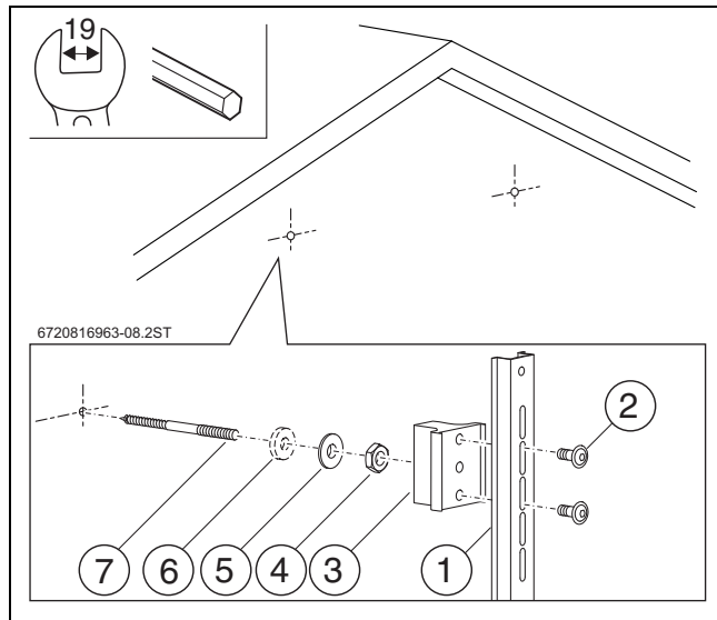
Bild 36 Profilschienen mit dem Stockschauben-Set montieren
