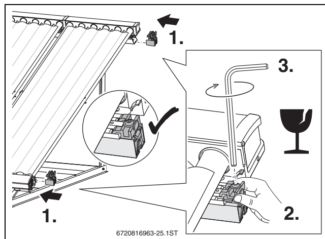
Bild 53 Kollektorspanner montieren
