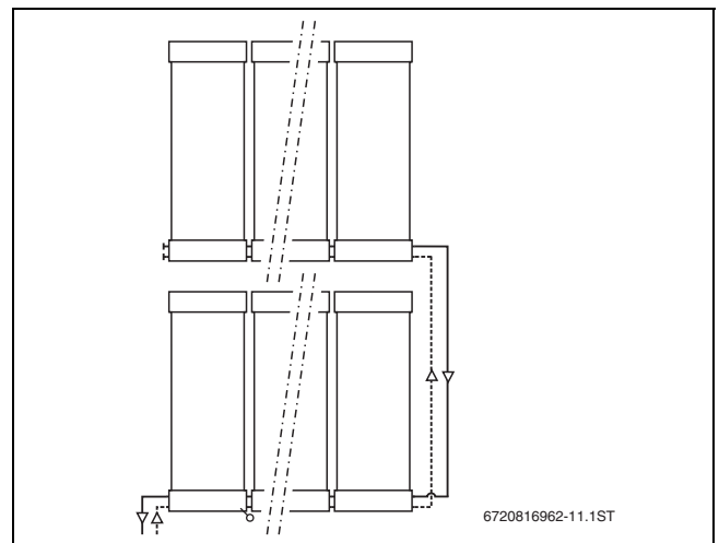
Bild 13 Maximal 7 Kollektoren, gleichseitiger Anschluss rechts oder links (2 Reihen)
