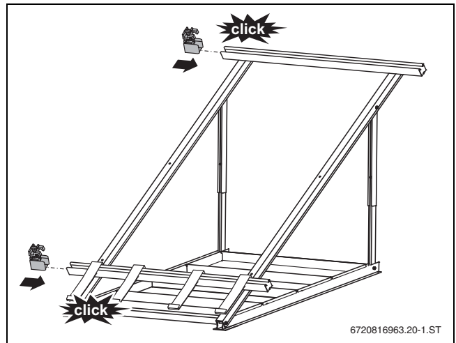
Bild 44 Kollektorspanner montieren
