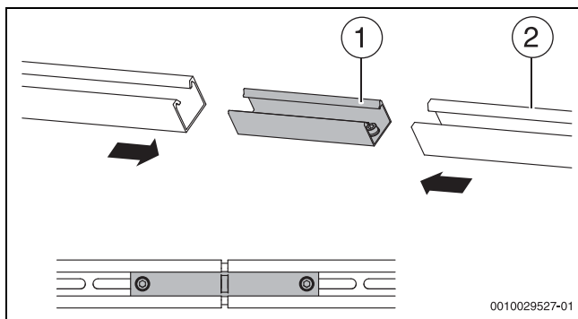
Bild 40 Profilschienen verbinden
