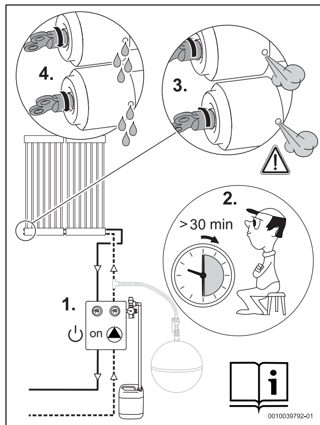
Bild 63 Entlüften
