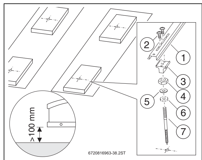
Bild 38 Profilschienen mit Stockschauben montieren
