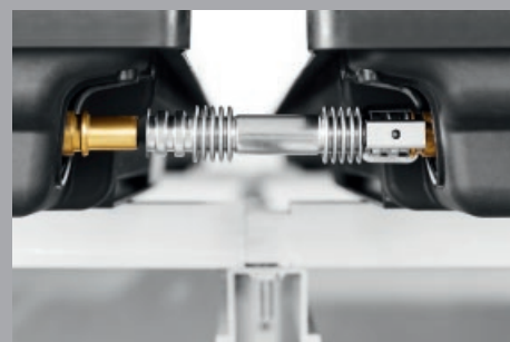
Edelstahl-Steckverbinder bei Logasol SKT 1.0.
