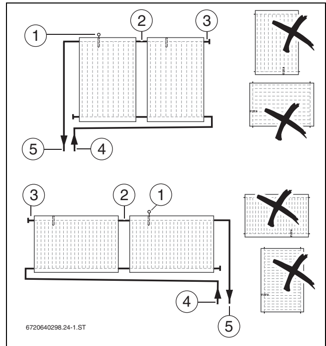
Bild 10 Anordnung senkrechter und waagerechter Kollektoren
