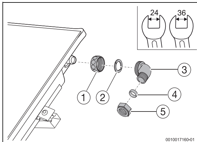
Bild 62 Winkeltülle montieren
