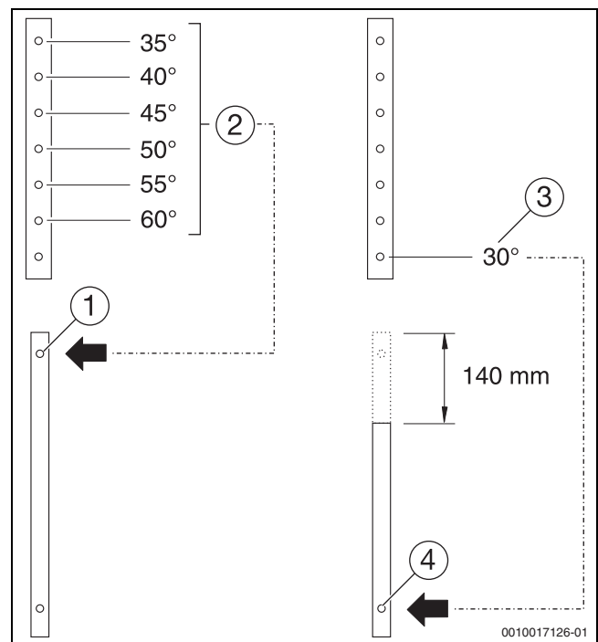
Bild 24 Teleskopschienen montieren - Kollektortyp waagerecht
