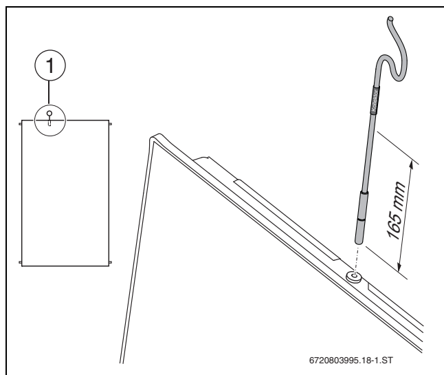
Bild 59 Kollektortemperaturfühler montieren
