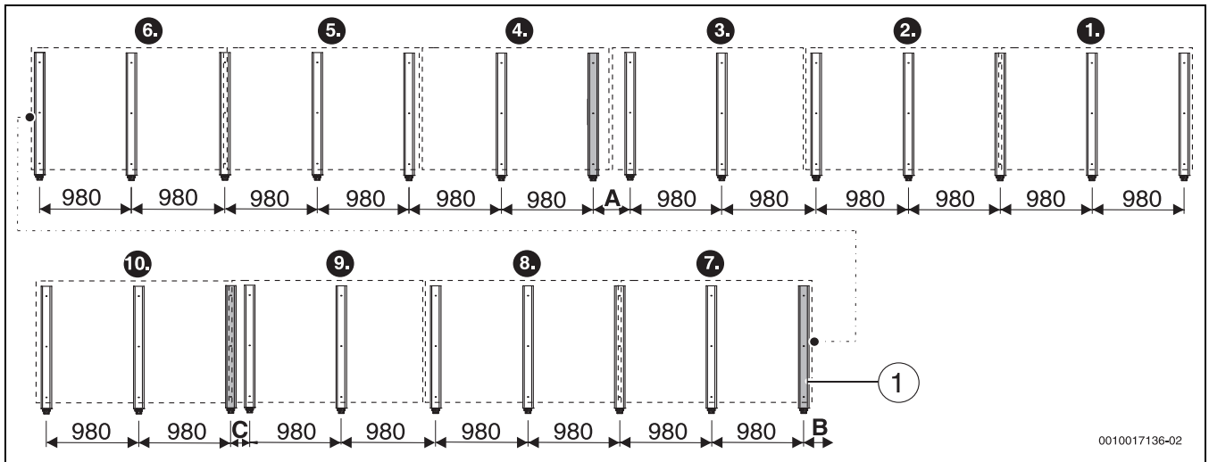
Bild 34 Grundaufführung Beschwerungswannen, 10 waagerechte Kollektoren (Angaben in mm)
