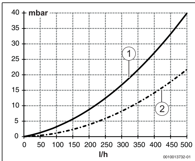
Bild 3 Druckverlustkurve (Wasser-Glykol-Gemisch)
