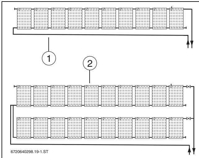
Bild 11 Hydraulischer Anschluss
