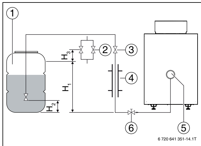
Bild 27 Installationsbeispiel
