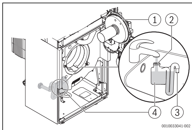
Bild 78 Siphon reinigen
