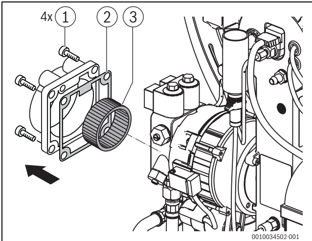
Bild 71 Ölpumpenfilter prüfen
