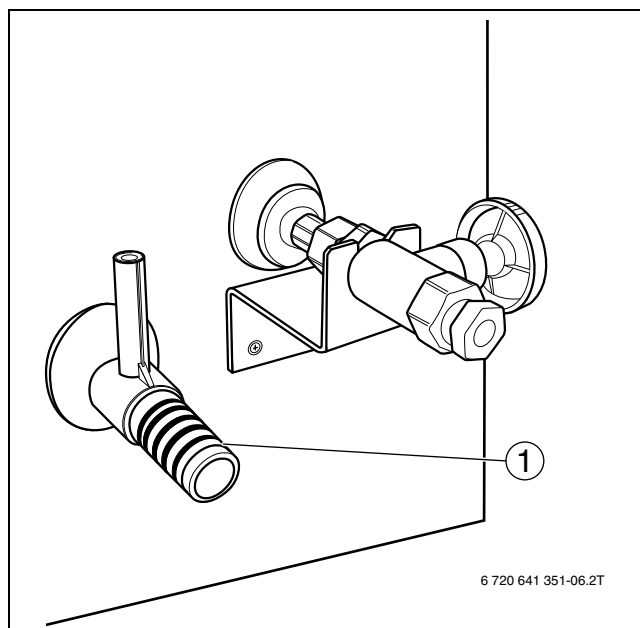
Bild 18 Anschluss Kondensatschlauch (dargestellt KB195i.2-19/25 BZ)
