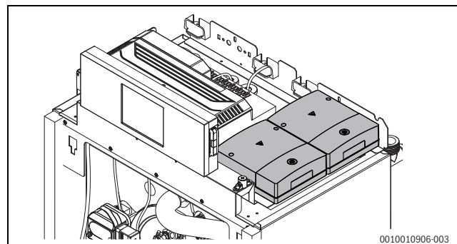
Bild 39 Standard-Funktionsmodule montiert
