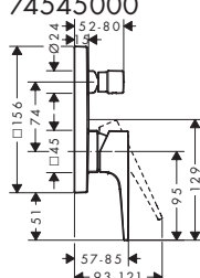
Metropol 32545XX0 / 74545000
